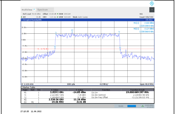
1-N7-PC3-15-20-M-3-CP-64QAM-Outer_Full-106@0-A nt1-19-19.560-≤20-PASS
