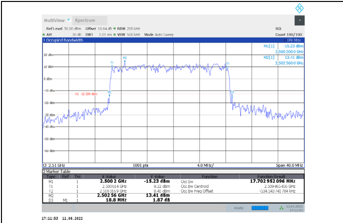
1-N7-PC3-15-20-L-7-DFT-16QAM-Outer_Full-100@0-A nt1-17.703-18.800-≤20-PASS
