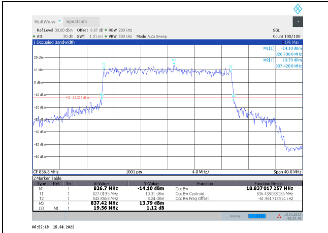
1-N5-PC3-15-20-M-3-CP-64QAM-Outer_Full-106@ 0-Ant1-18.837-19.560-≤20-PASS
