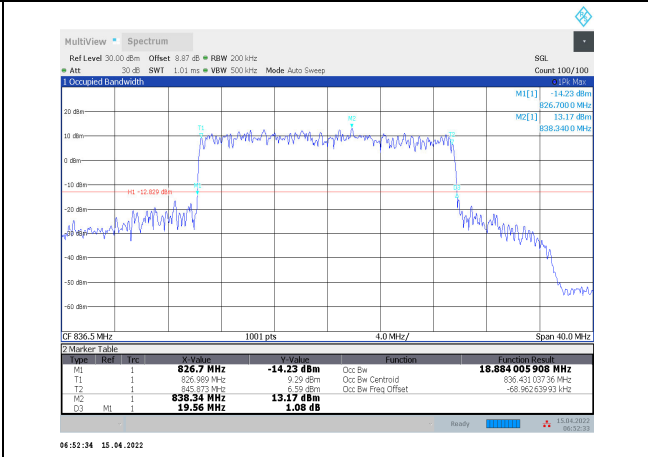
1-N5-PC3-15-20-M-2-CP-16QAM-Outer_Full-106@ 0-Ant1-18.884-19.560-≤20-PASS
