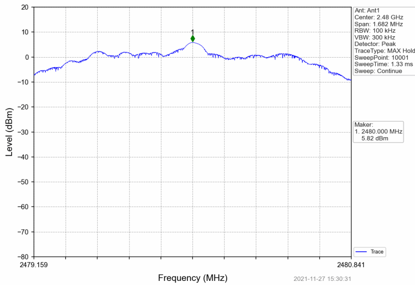
2M_HCH_2480MHz_DataRate=_Ant1_NTNV
