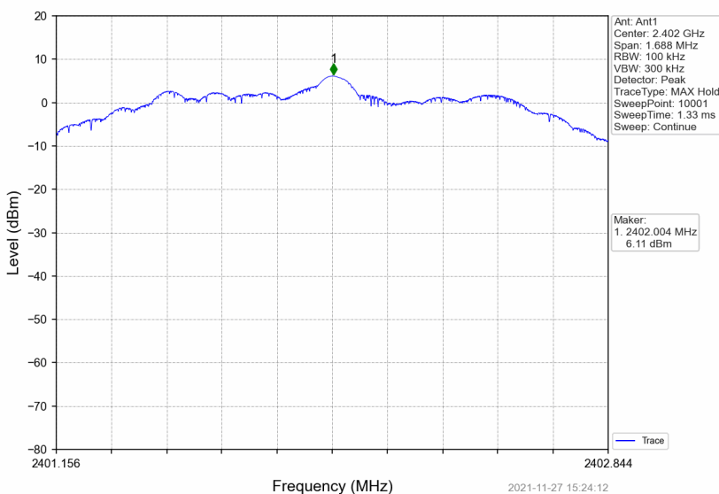
2M_LCH_2402MHz_DataRate=_Ant1_NTNV
