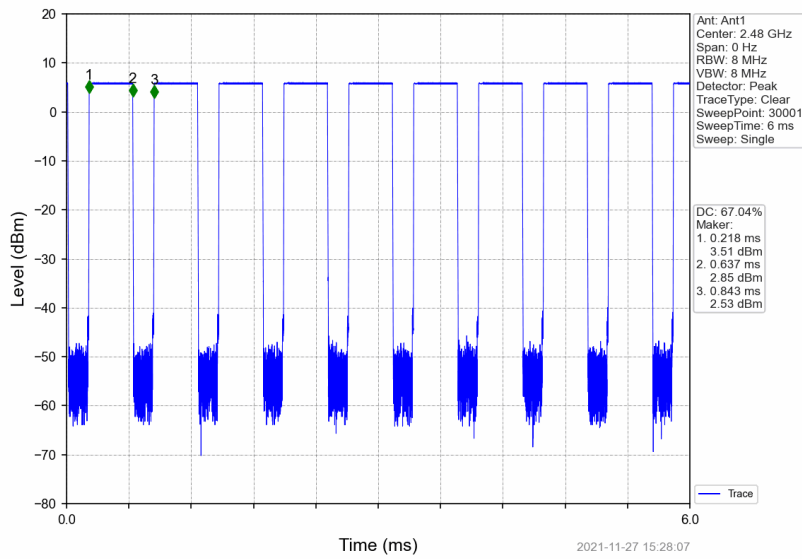
1M_HCH_2480MHz_DataRate=_Ant1_NTNV
