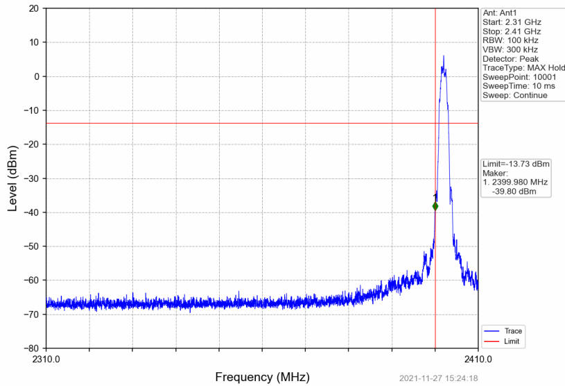
2M_LCH_2402MHz_DataRate=_Ant1_NTNV
