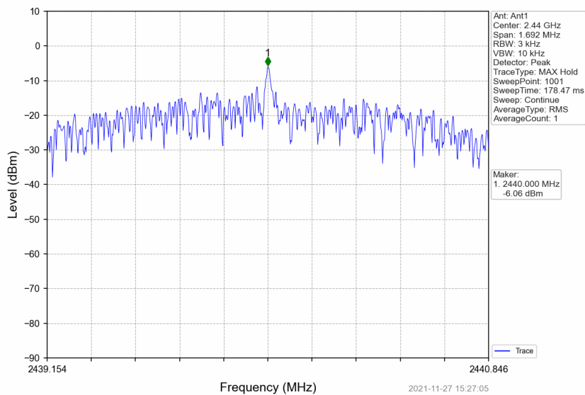
2M_MCH_2440MHz_DataRate=_ Ant1_NTNV
