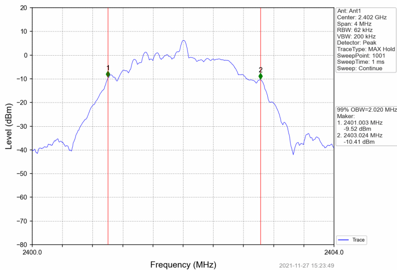
2M_LCH_2402MHz_DataRate=_Ant1_NTNV
