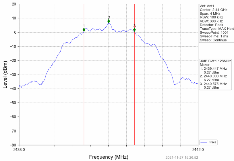
2M_MCH_2440MHz_DataRate=_Ant1_NTNV
