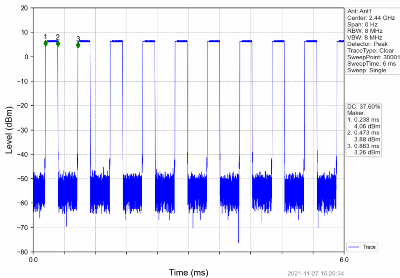
2M_MCH_2440MHz_DataRate=_ Ant1_NTNV
