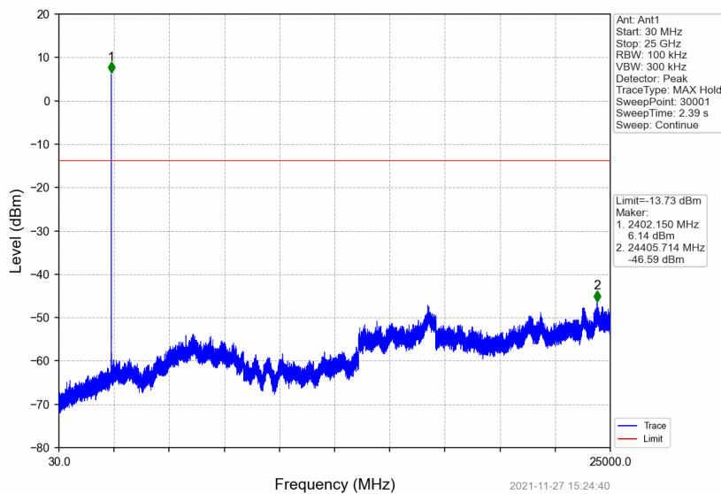
2M_LCH_2402MHz_DataRate=_Ant1_NTNV
