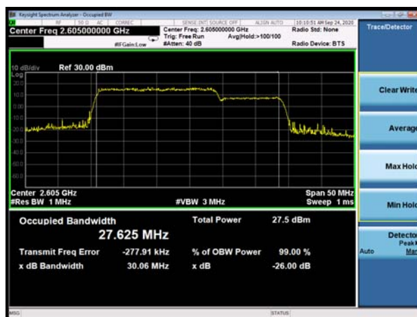
CA_41C 64QAM 20MHz+10MHz
