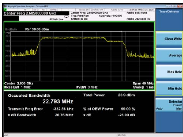
CA_41C_64QAM_20MHz+5MHz
