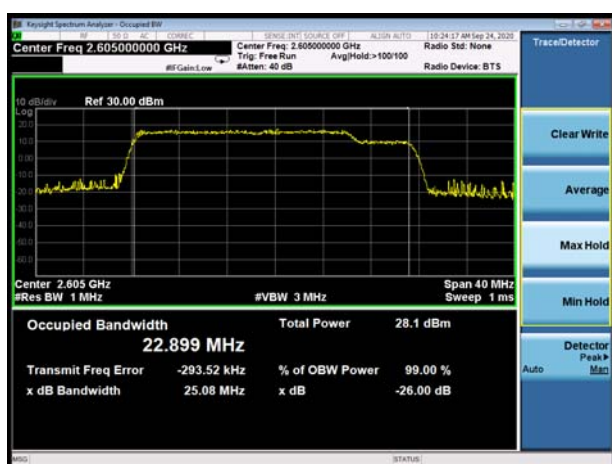
CA_41C_64QAM_20MHz+5MHz
