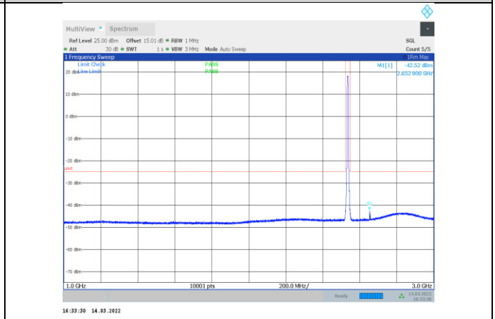
1-N7-PC3-15-5-M-3-CP-QPSK-Outer_Full-25@0-1000-3 000-Ant1--42.52--25-PASS
