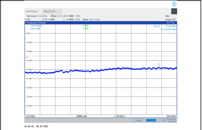
1-N7-PC3-15-15-L-3-CP-QPSK-Outter_Full-79@0-12000 -26900-Ant1--37.09--25-PASS
