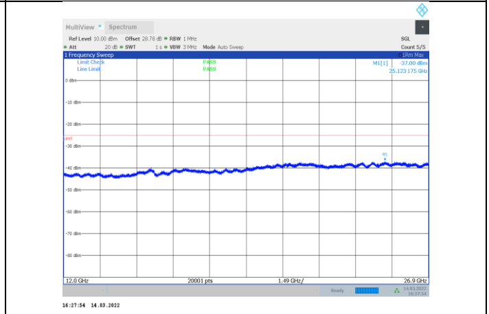
1-N7-PC3-15-5-L-2-CP-QPSK-Edge_1RB_Right-1@24 -12000-26900-Ant1--37.00--25-PASS
