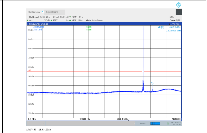
1-N7-PC3-15-5-L-2-CP-QPSK-Edge_1RB_Right-1@24 -1000-3000-Ant1--40.35--25-PASS
