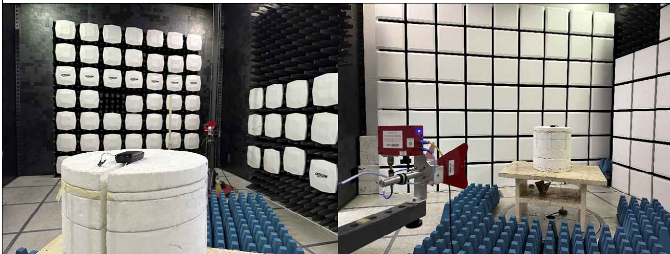
3GHz – 18GHz
