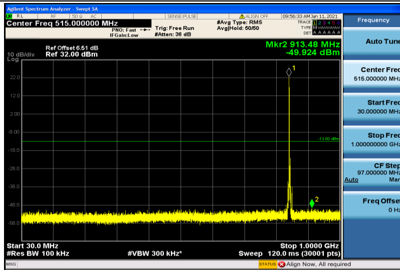
Band26-5MHz-QPSK-27015-1RB#0-30~1000MHz
