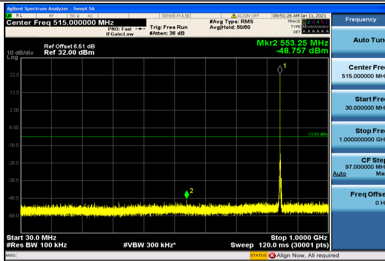
Band26-3MHz-QPSK-27025-1RB#0-30~1000MHz
