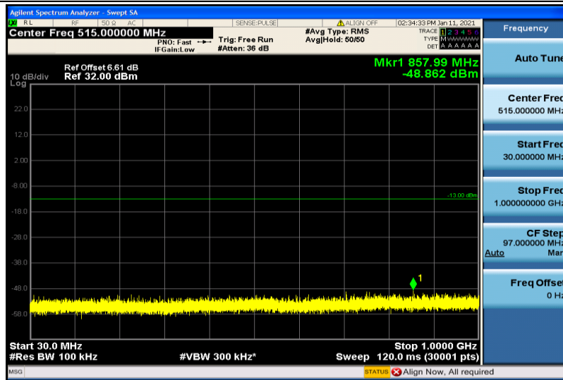
Band25-20MHz-QPSK-26590-1RB#0-30~1000MHz
