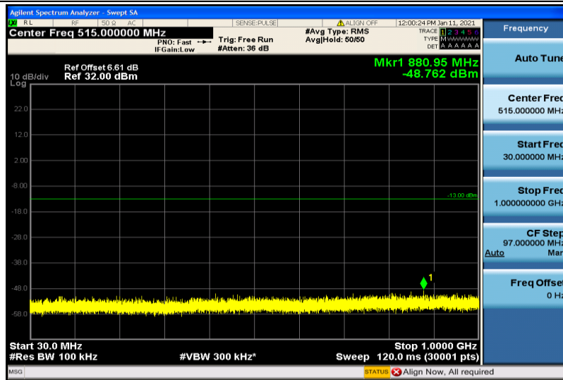
Band2-20MHz-16QAM-18900-1RB#0-30~1000MHz
