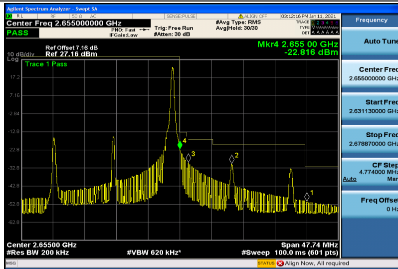
Band41-20MHz-QPSK-41140-1RB#99
