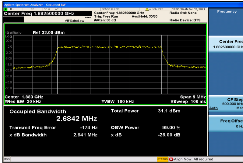
Band25-3MHz-QPSK-26365-15RB#0-2.6842
