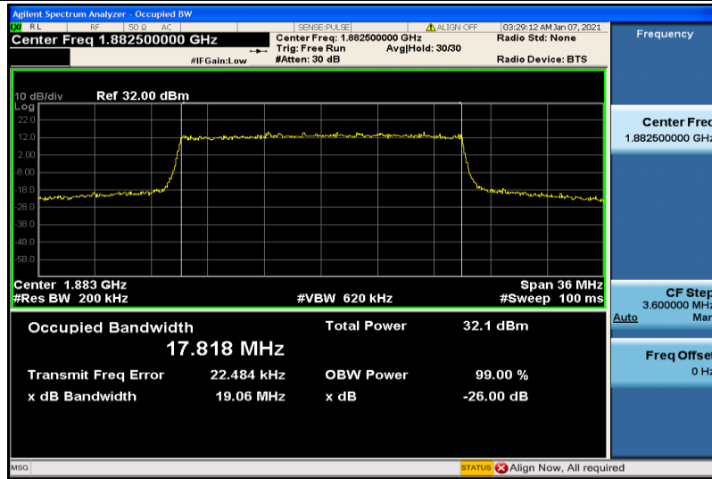
Band25-20MHz-QPSK-26365-100RB#0-17.818
