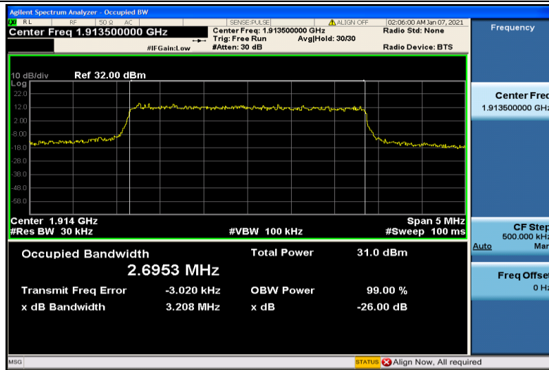
Band25-3MHz-QPSK-26675-15RB#0-2.6953
