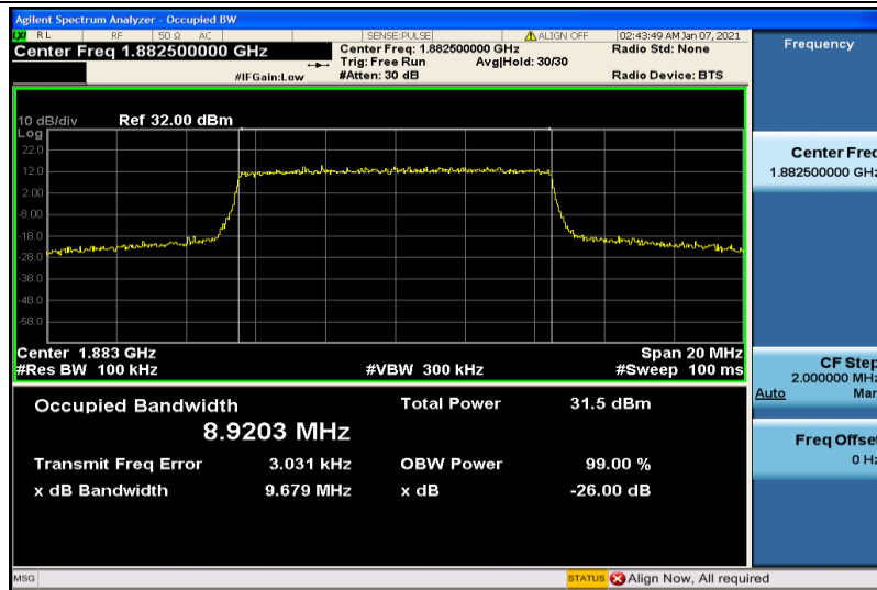
Band25-10MHz-QPSK-26365-50RB#0-8.9203
