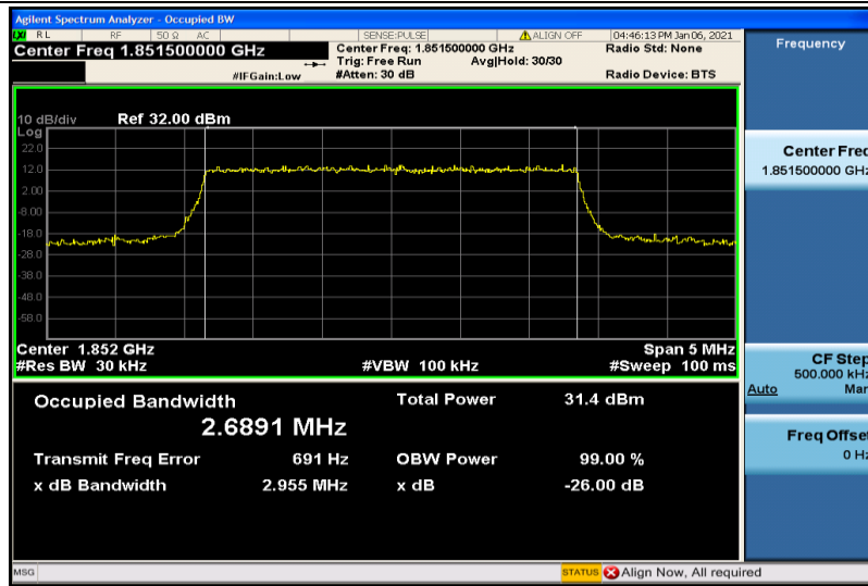
Band2-3MHz-QPSK-18615-15RB#0-2.6891
