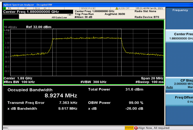
Band2-10MHz-QPSK-18900-50RB#0-8.9274
