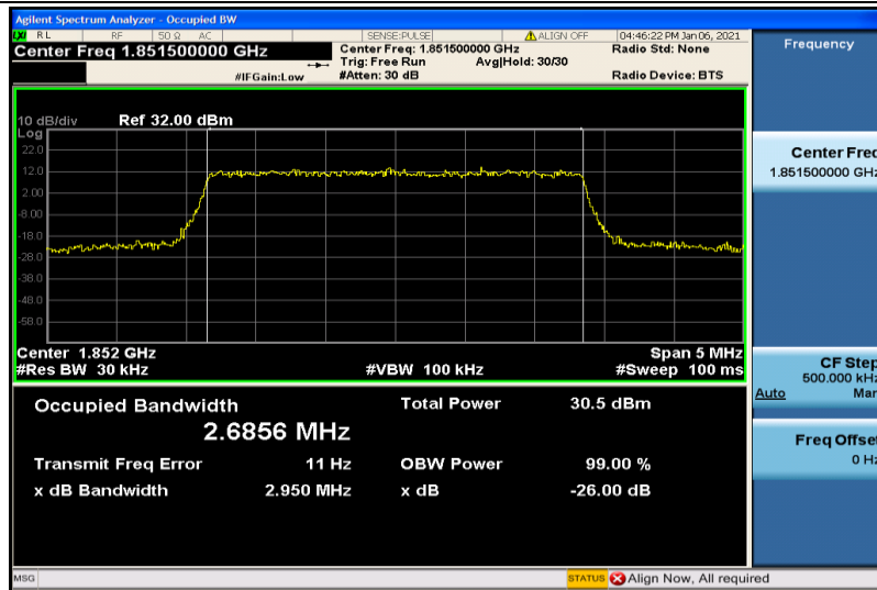
Band2-3MHz-16QAM-18615-15RB#0-2.6856
