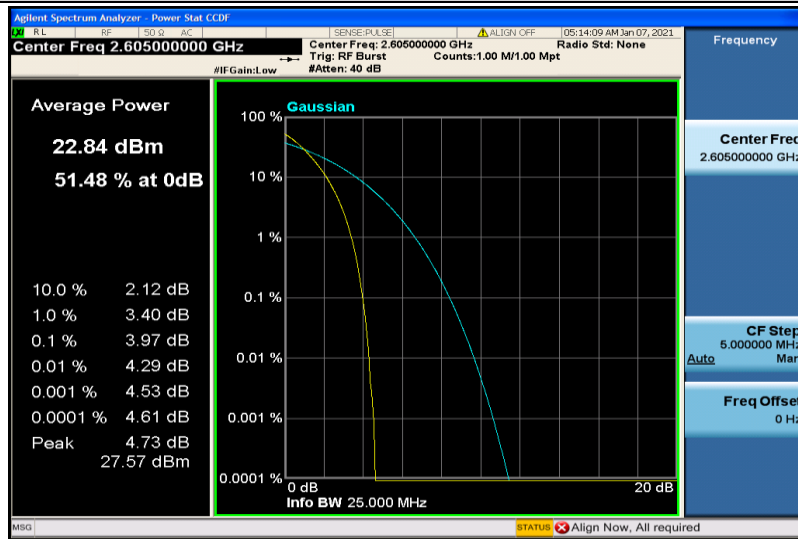
Band41-20MHz-QPSK-40740-100RB#0
