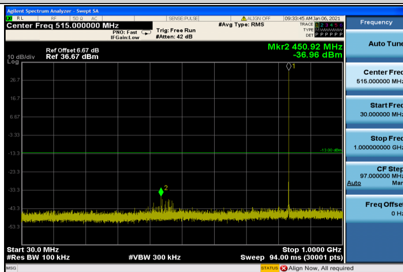
GSM850-190-30~1000
