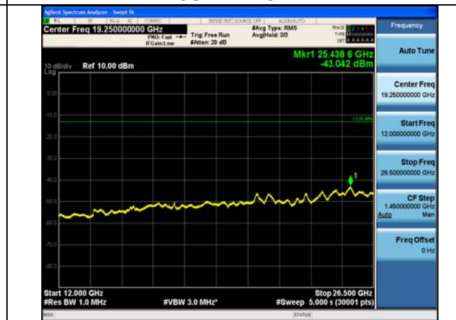
12GHz ~26.5GHz
