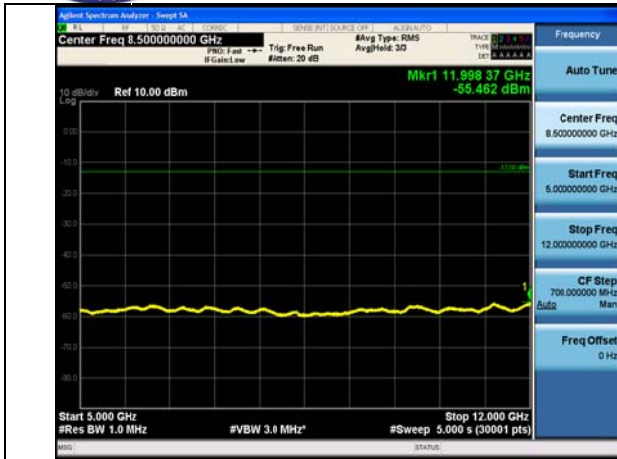
5GHz ~12GHz
