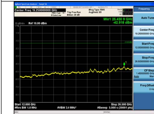
12GHz ~26.5GHz
