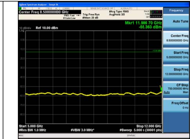
5GHz ~12GHz
