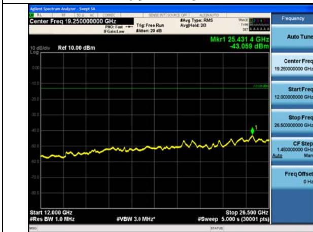
12GHz ~26.5GHz
