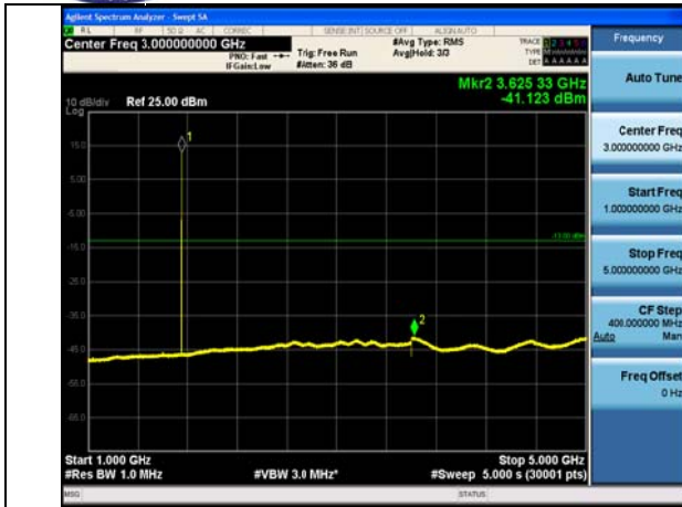
1GHz ~5GHz
