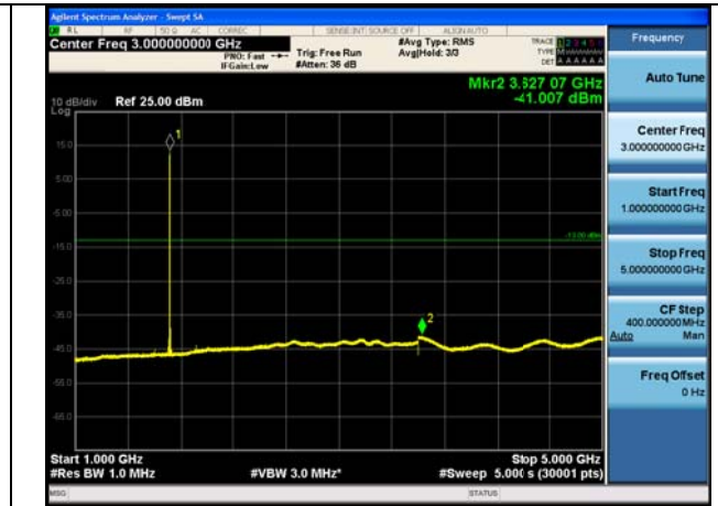
1GHz ~5GHz
