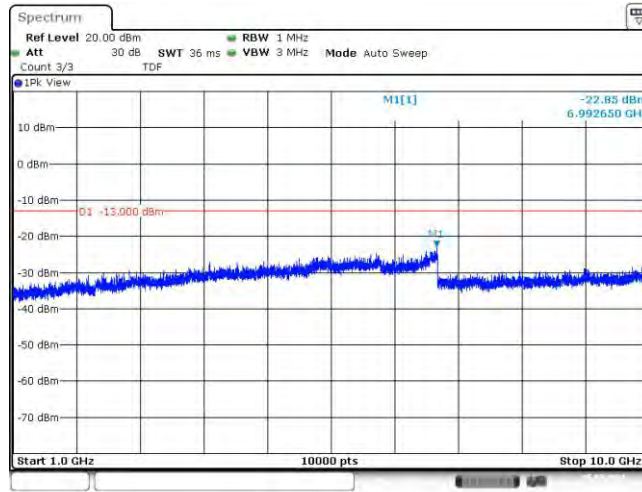
Band26-1.4MHz-QPSK-26797-6RB#0-Range2:1000~10000MHz
