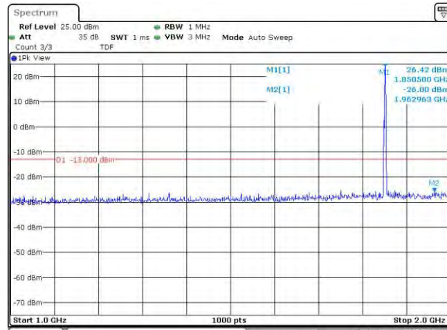
Band25-1.4MHz-QPSK-26047-1RB#0-Range2:1000~2000MHz
