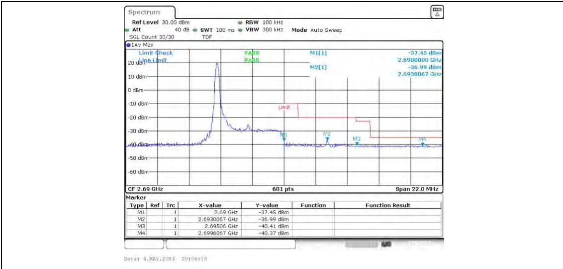
Band41-5MHz-16QAM-41565-1RB#24
