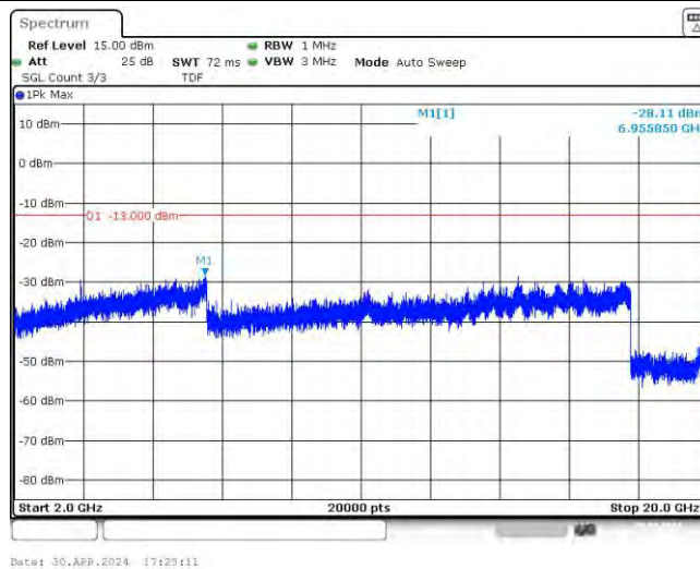
Band25-1.4MHz-QPSK-26047-6RB#0-Range3:2000~20000MHz
