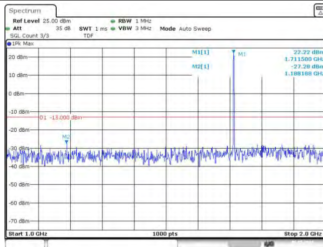
Band4-1.4MHz-QPSK-19957-6RB#0-Range2:1000~2000MHz
