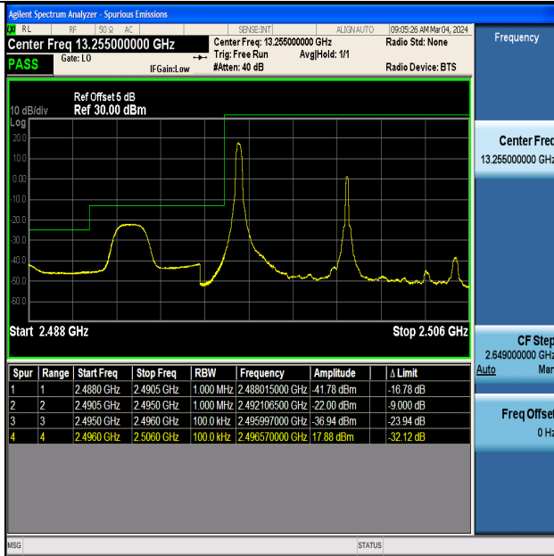
Band41_10MHz_QPSK_39700_1RB#0
