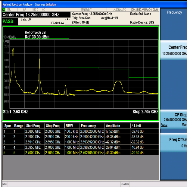
Band41_10MHz_QPSK_41540_1RB#0
