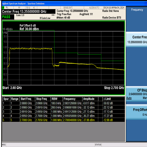
Band41_10MHz_QPSK_41540_50RB#0
