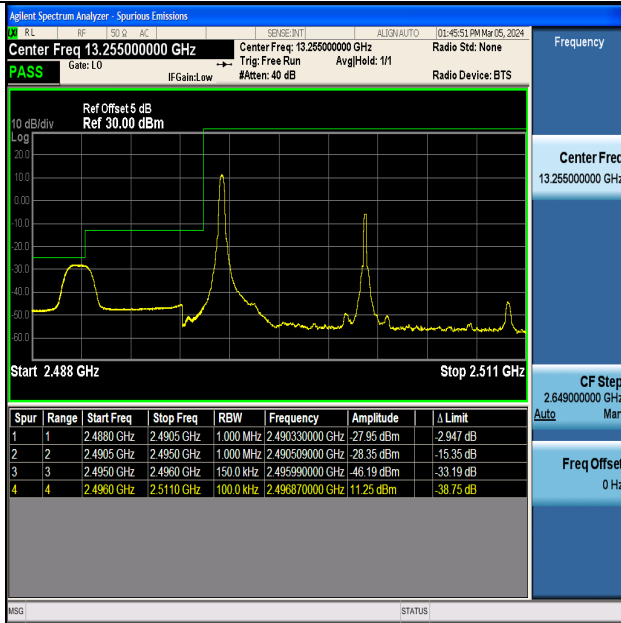
Band41_15MHz_QPSK_39725_1RB#0
