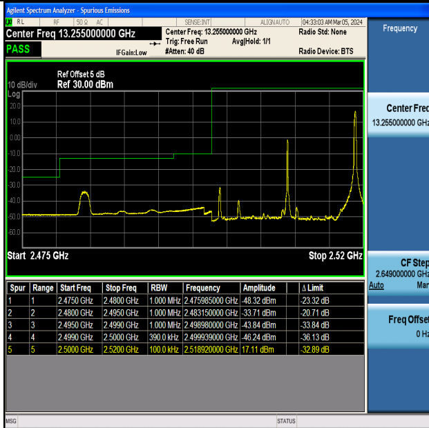
Band7_20MHz_16QAM_20850_1RB#99
