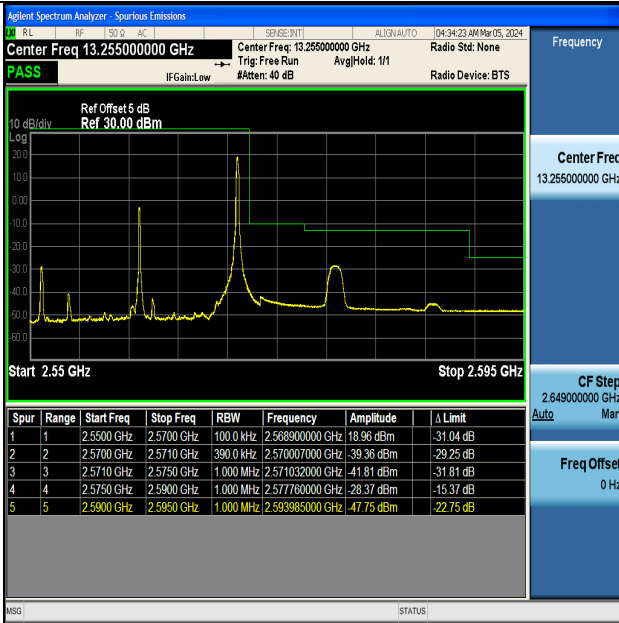
Band7_20MHz_QPSK_21350_1RB#99
