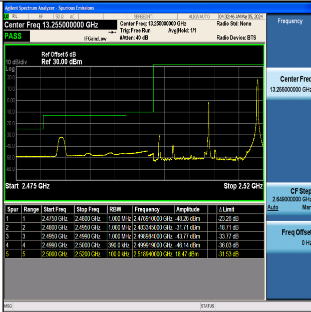
Band7_20MHz_QPSK_20850_1RB#99
