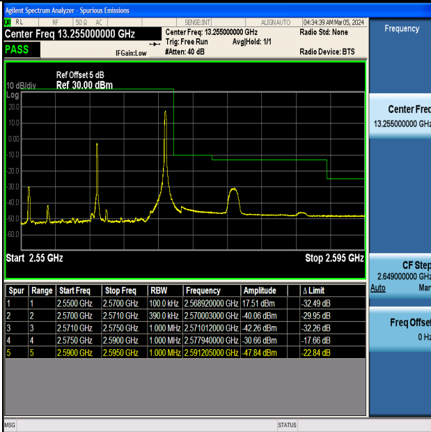
Band7_20MHz_16QAM_21350_1RB#99
