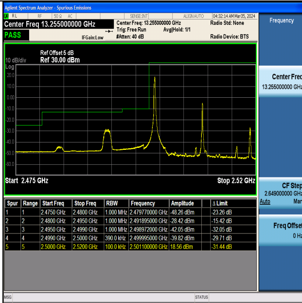
Band7_20MHz_QPSK_20850_1RB#0
