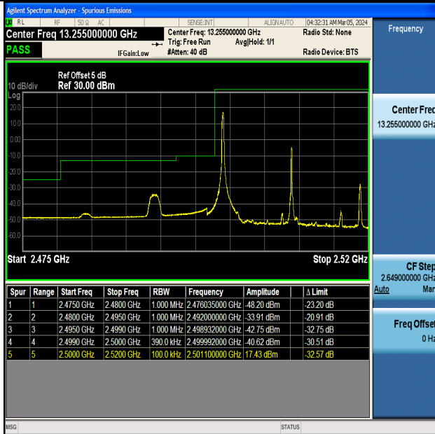
Band7_20MHz_16QAM_20850_1RB#0
