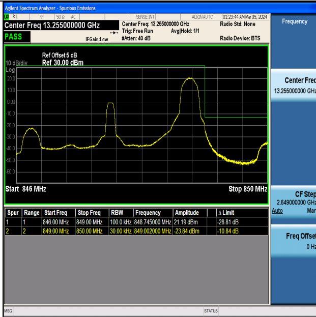
Band5_3MHz_QPSK_20635_1RB#14
