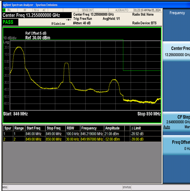
Band5_3MHz_QPSK_20635_1RB#0
