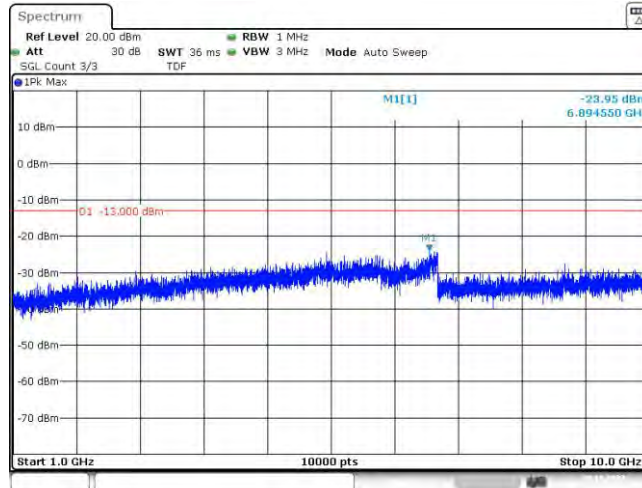
Band26-1.4MHz-QPSK-26797-6RB#0-Range2:1000~10000MHz
