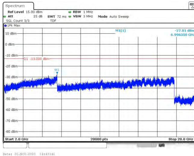
Band25-1.4MHz-QPSK-26047-6RB#0-Range3:2000~20000MHz
