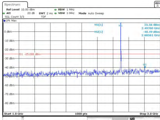
Band41-5MHz-QPSK-39675-1RB#0-Range2:1000~3000MHz
