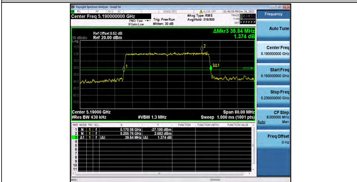
11AX40SISO_Ant1_5190
