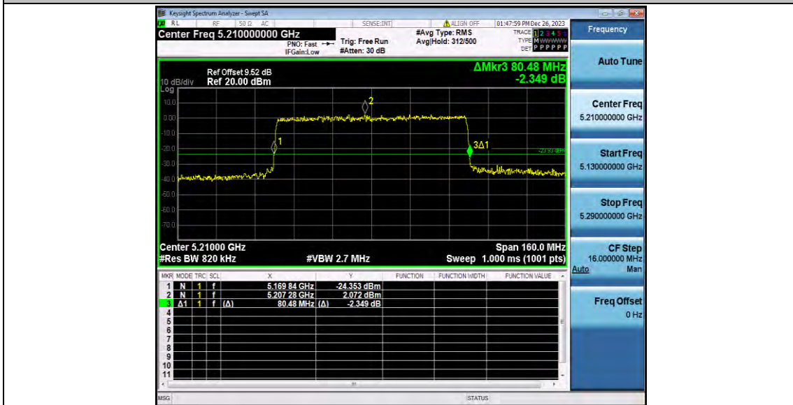
11AX80SISO_Ant1_5210
