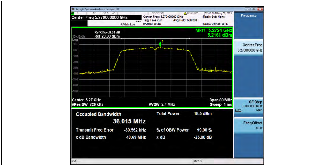
11AX40SISO_Ant1_5270
