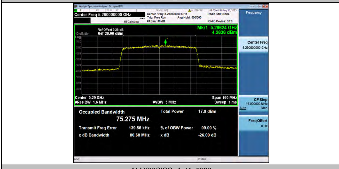
11AX80SISO_Ant1_5290
