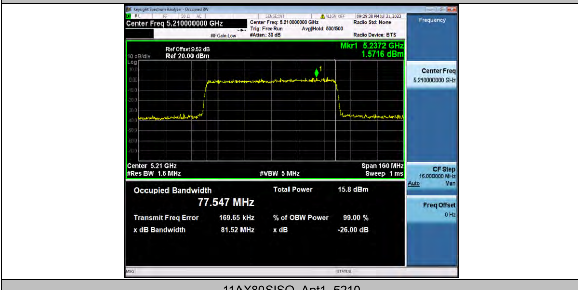
11AX80SISO_Ant1_5210
