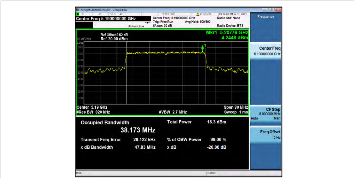
11AX40SISO_Ant1_5190
