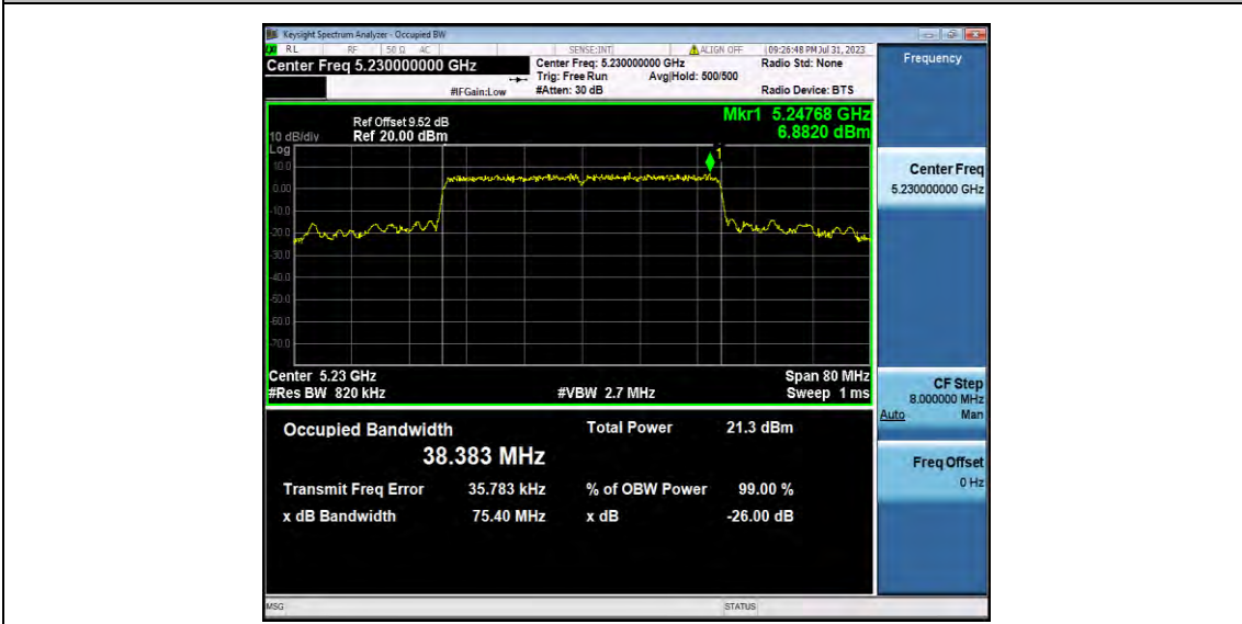
11AX40SISO_Ant1_5230
