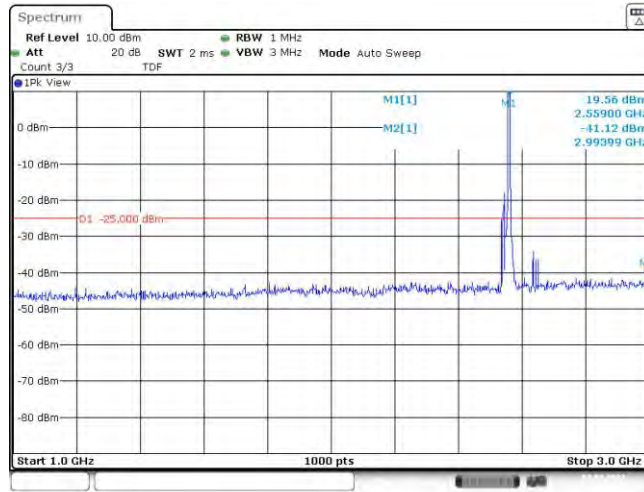
Band41-5MHz-QPSK-40265-25RB#0-Range2:1000~3000MHz
