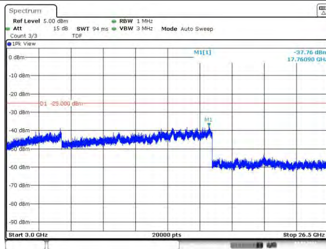
Band41-5MHz-QPSK-40265-25RB#0-Range3:3000~26500MHz
