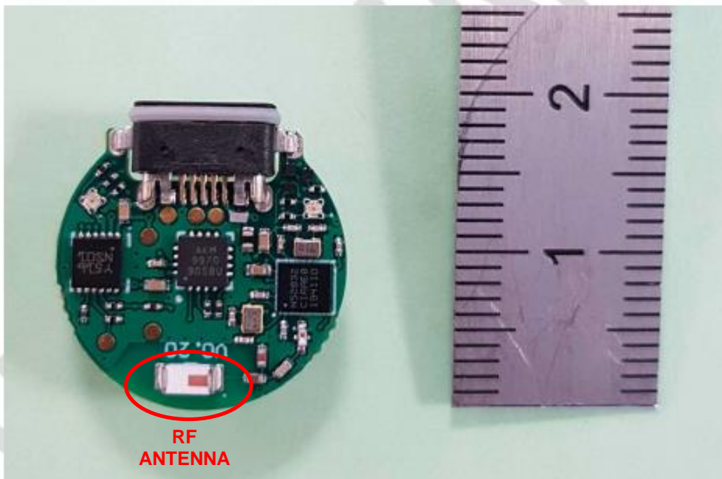
Figure 2 – SoloSmart Mini – ILO PCB bottom
