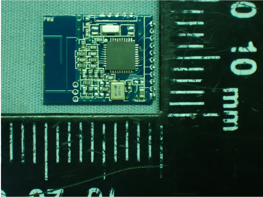
Figure 17 BLE Module, Front View
