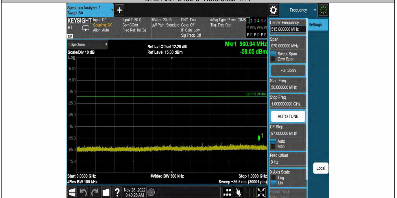
DH5-Ant1-2402-30~1000-1.11
