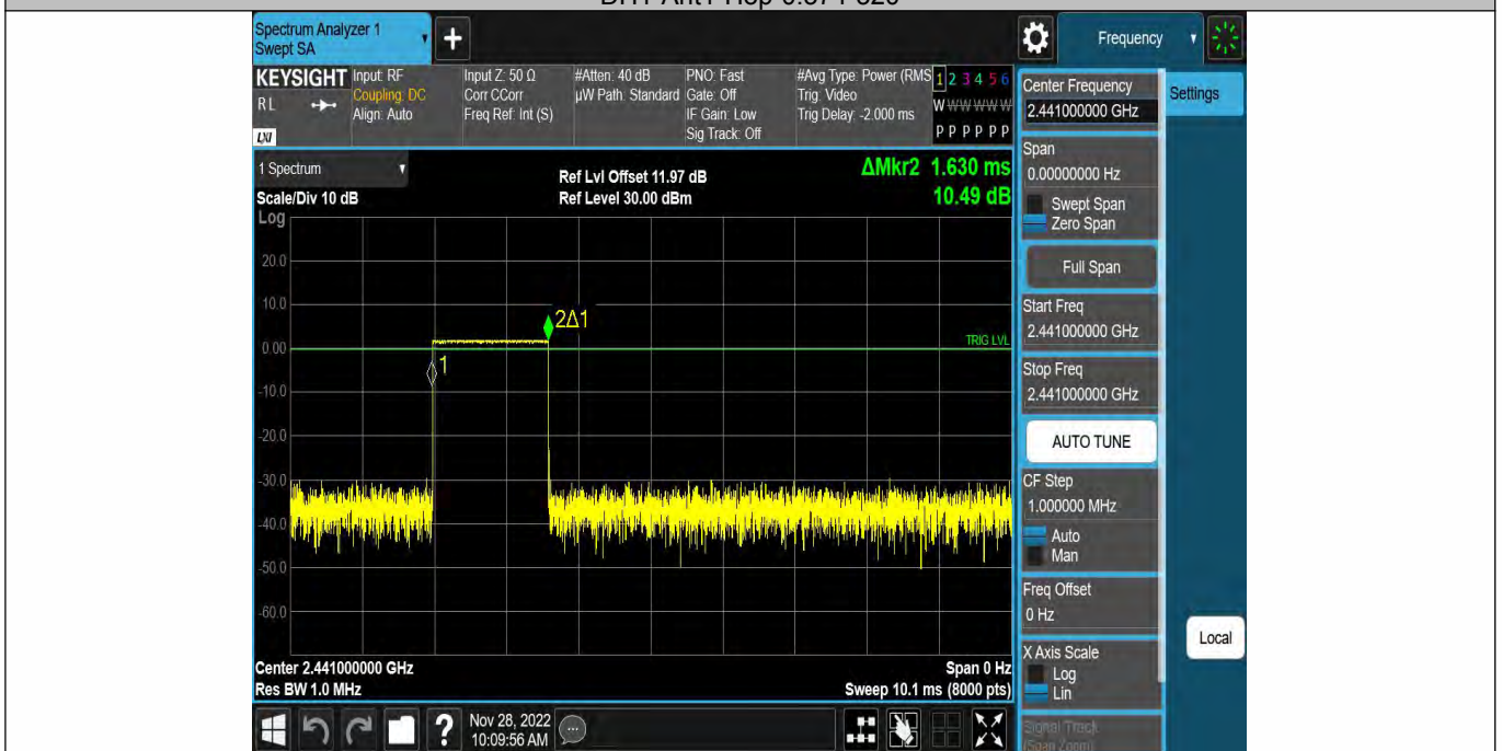
DH3-Ant1-Hop-1.630-160
