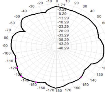
2450.0MHz Total(E1-XZ), Max= 0.45dBi
