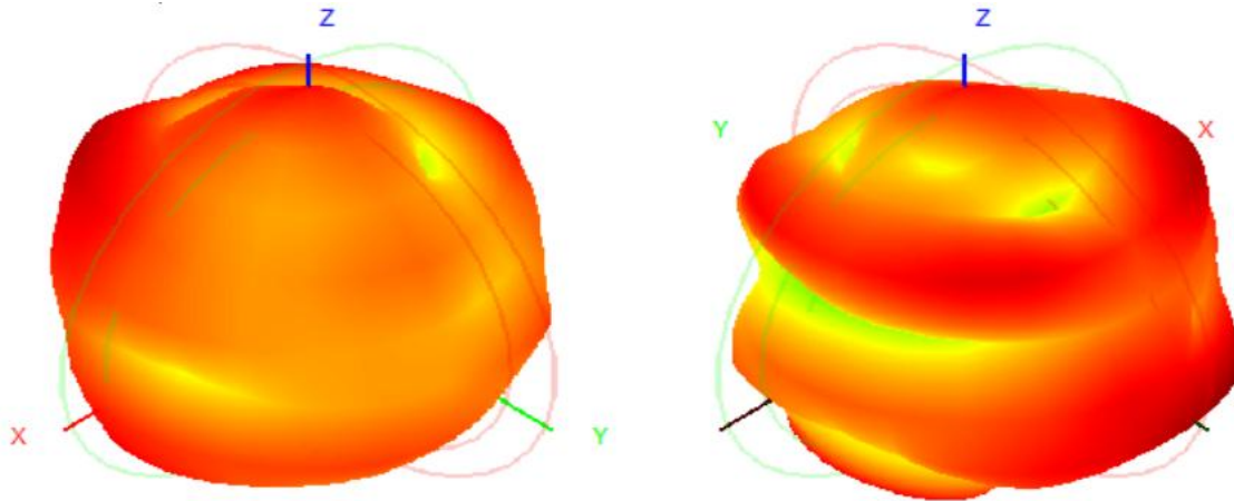
2450.0MHz Total(E2-YZ), Max= 0.98dBi
