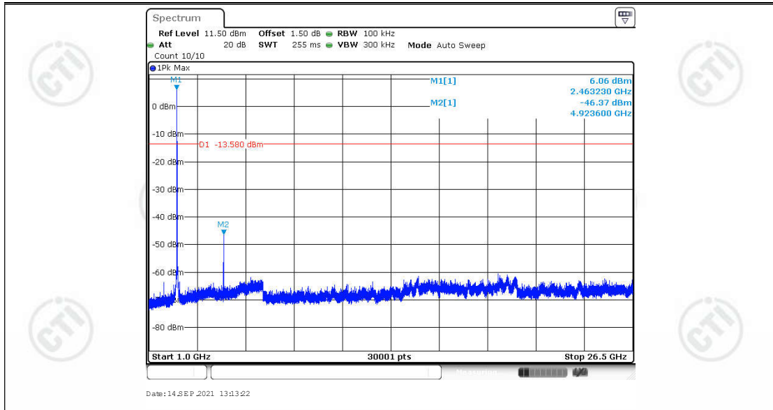
11B_Ant1_2462_1000~26500
