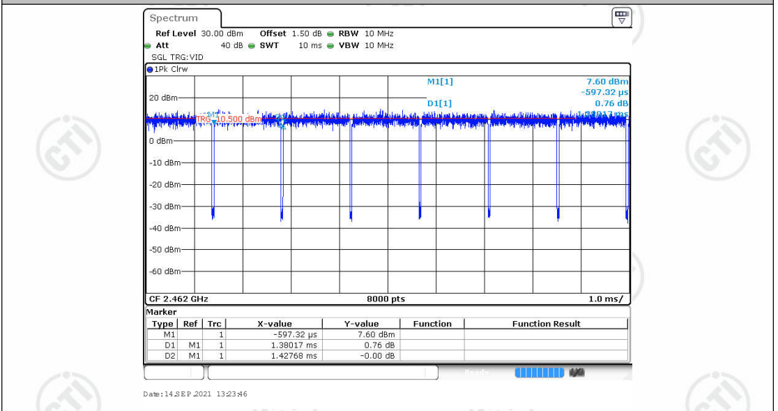
11G_Ant1_2462
