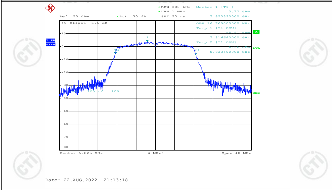
11A_Ant1_5825
