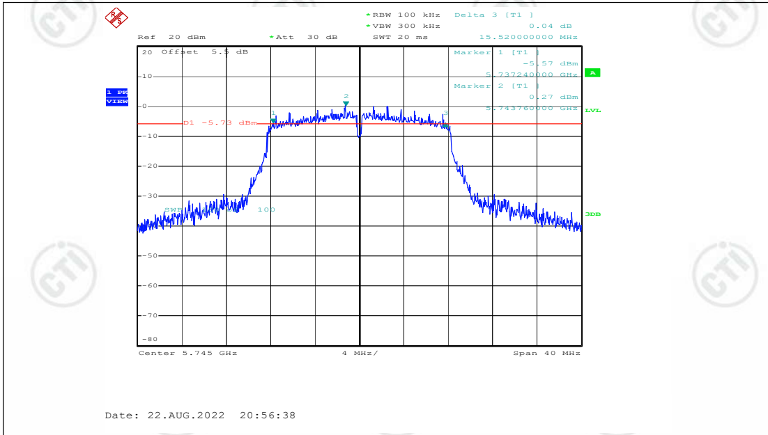
11A_Ant1_5745
