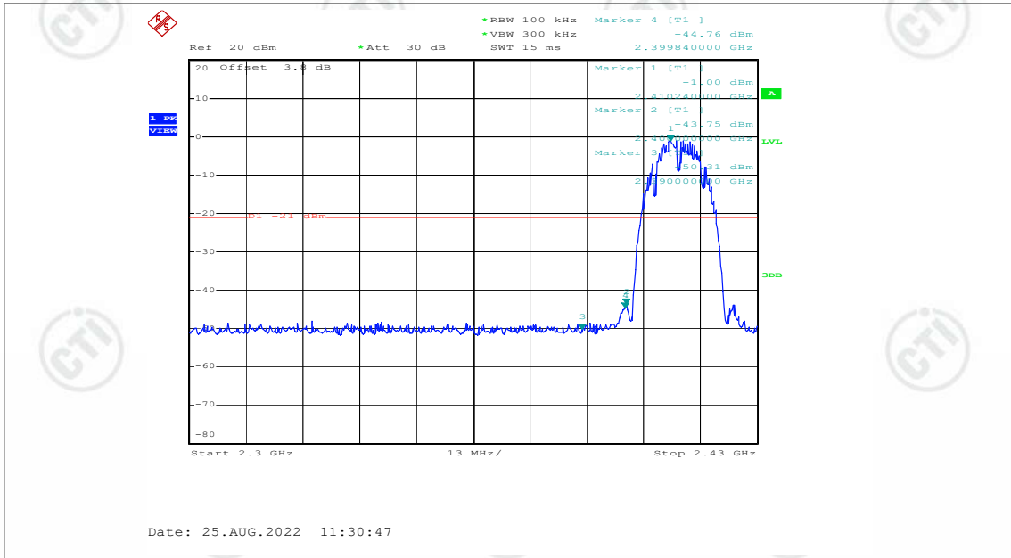
11B_Ant1_Low_2412
