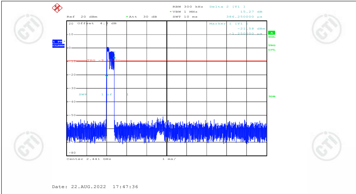
2DH1_Ant1_Hop
