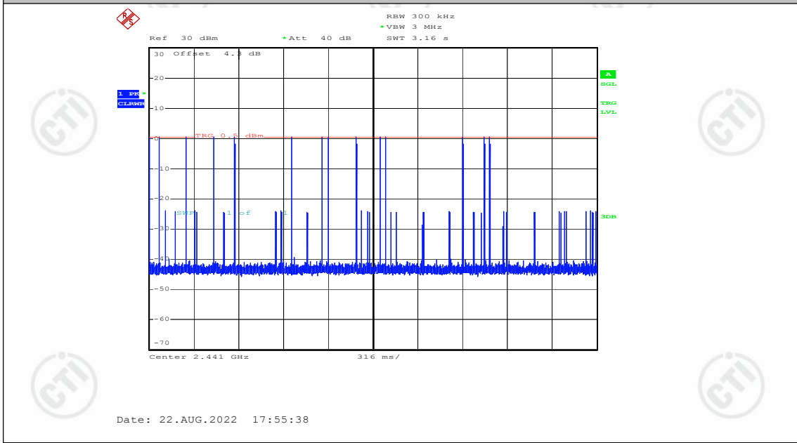
3DH3_Ant1_Hop
