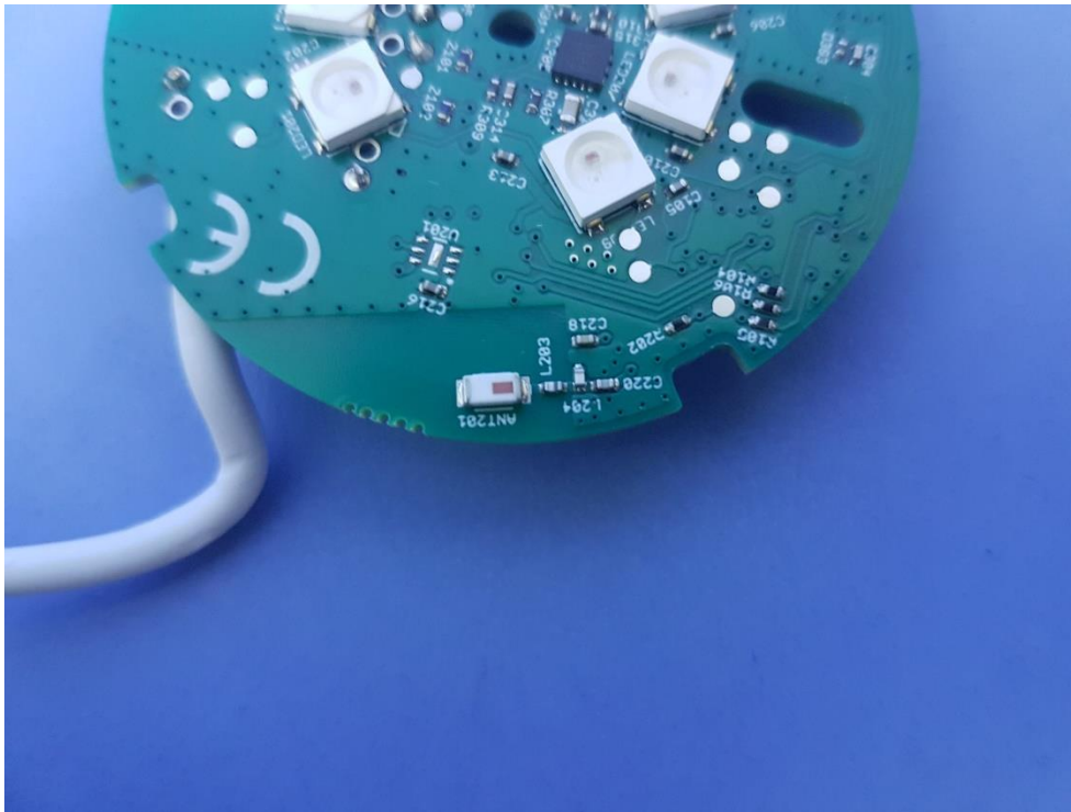
BLE Antenna
