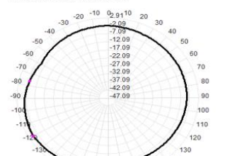
2470.0MHz Total(H), Max= 0.74dBi
