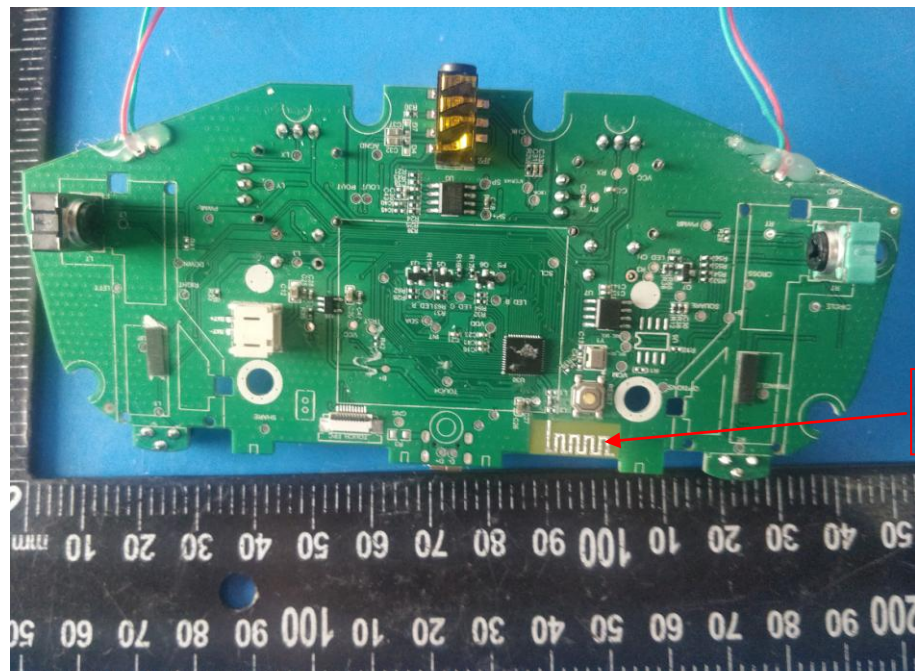
Antenna
