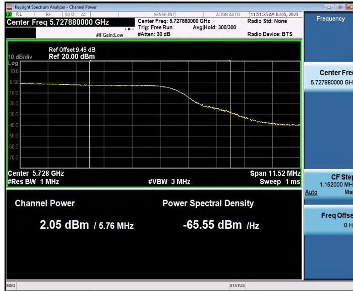
11A_Ant1_5720_UNII-3
