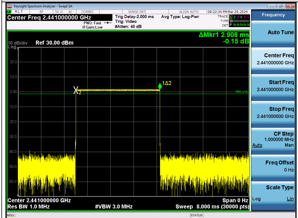
Test_Graph_BR_HOP_Chain A_NA_1Mbps_2441_Time per Burst
