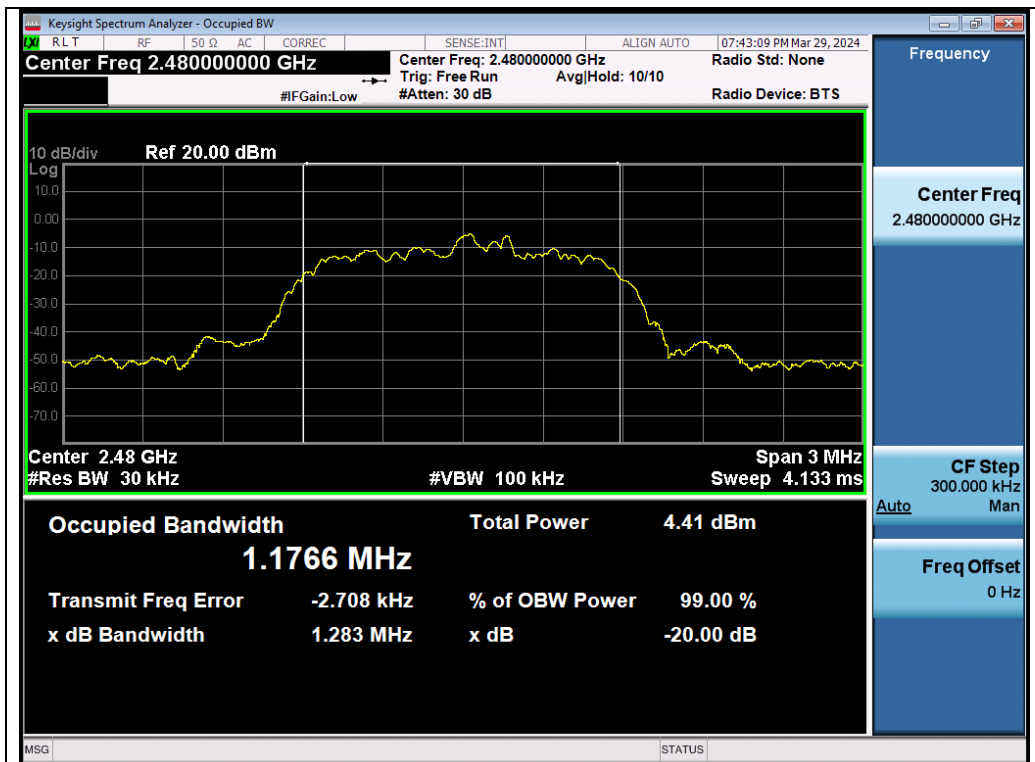
Test_Graph_EDR_Chain A_2480_2Mbps_OBW
