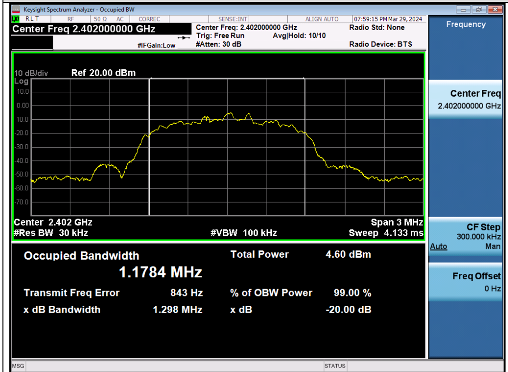
Test_Graph_EDR_Chain A_2402_3Mbps_OBW
