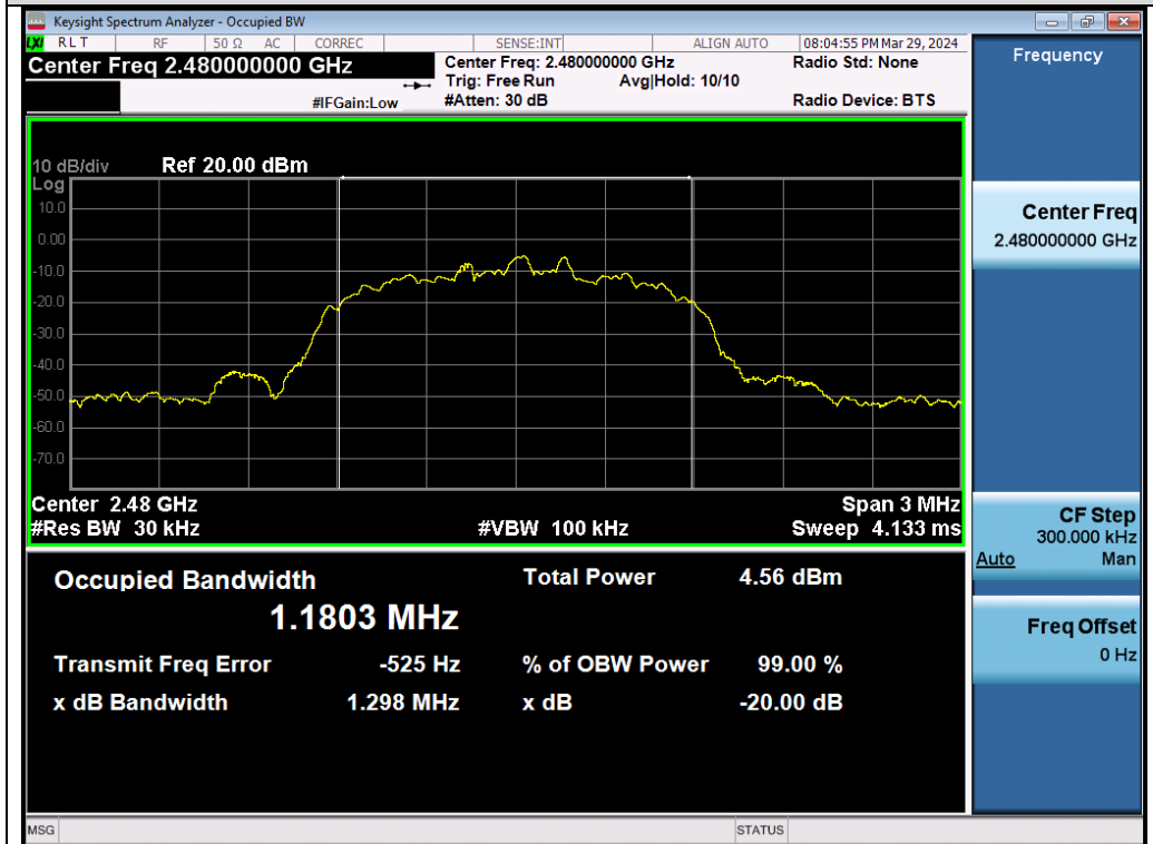
Test_Graph_EDR_Chain A_2480_3Mbps_OBW
