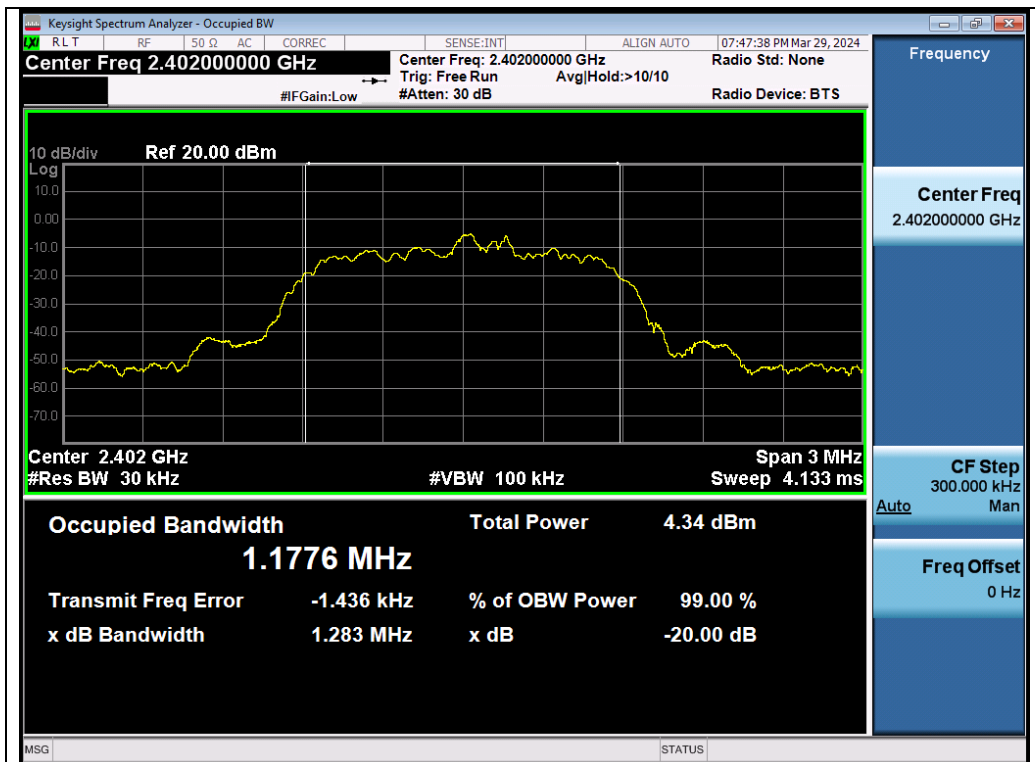
Test_Graph_EDR_Chain A_2402_2Mbps_OBW
