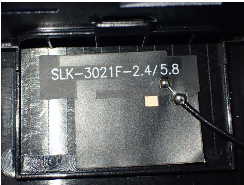
2.4GWIFI&5GWIFI ANTENNA
