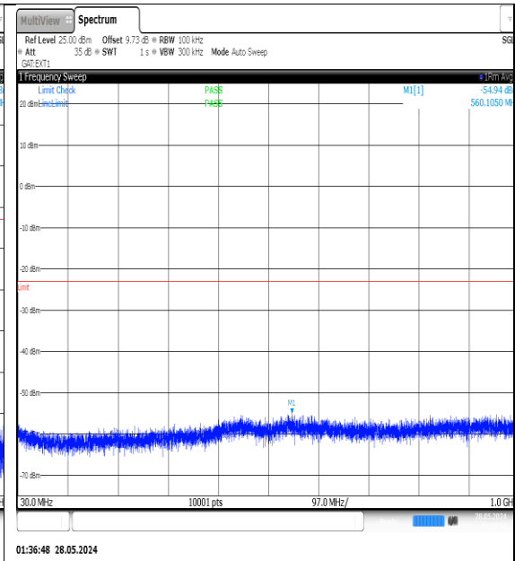
NTNV-N77-3450-3550-PC3-30-20-M-DFT-QPSK-Edge_1RB_Left-30-1000-Ant1-PASS
