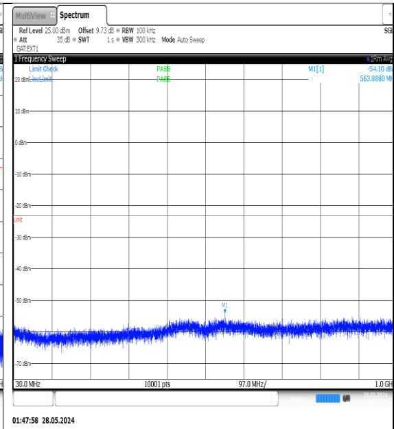
NTNV-N77-3450-3550-PC3-30-25-H-DFT-QPSK- Edge_1RB_Left-30-1000-Ant1-PASS
