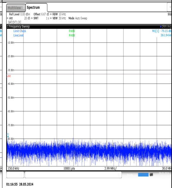
NTV-N77-3450-3550-PC3-30-10-L-DFT-QPSK- Edge_1RB_Left-0.15-30-Ant1-PASS
