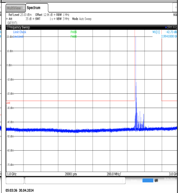
NTVN-N41-PC3-30-100-L-DFT-QPSK- Edge_1RB_Left-1000-3000-Ant1-PASS
