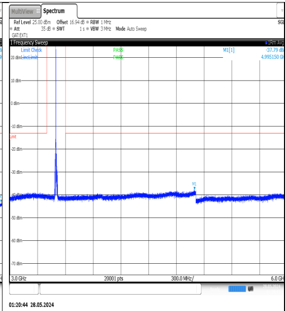
NTNV-N77-3450-3550-PC3-30-10-M-DFT-QPSK-Edge_1RB_Left-3000-6000-Ant1-PASS
