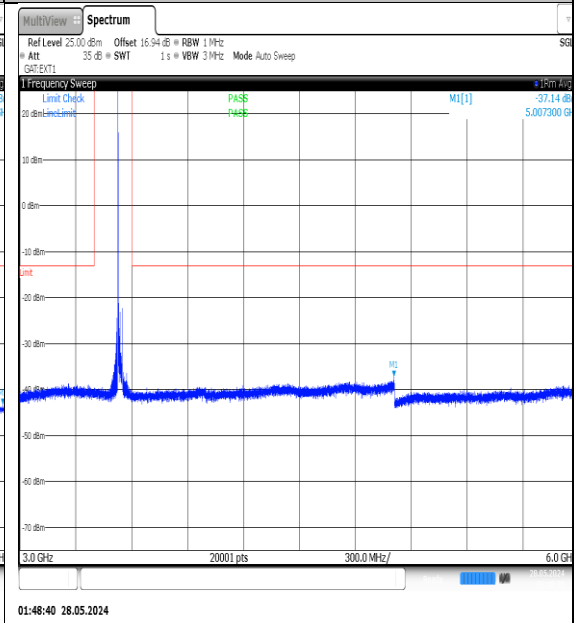
NTNV-N77-3450-3550-PC3-30-25-H-DFT-QPSK- Edge_1RB_Left-3000-6000-Ant1-PASS
