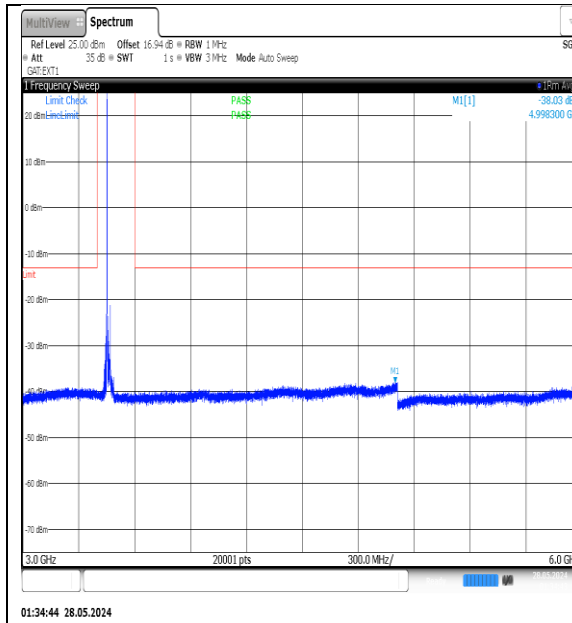
NTNV-N77-3450-3550-PC3-30-20-L-DFT-QPSK- Edge_1RB_Left-3000-6000-Ant1-PASS
