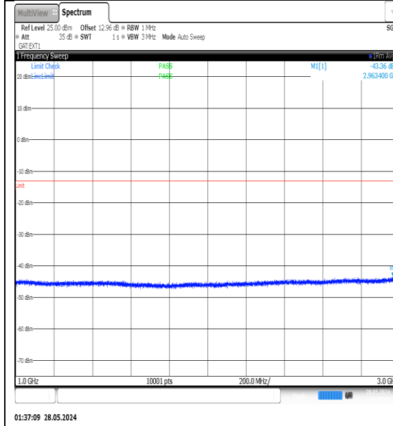
NTNV-N77-3450-3550-PC3-30-20-M-DFT-QPSK-Edge_1RB_Left-1000-3000-Ant1-PASS
