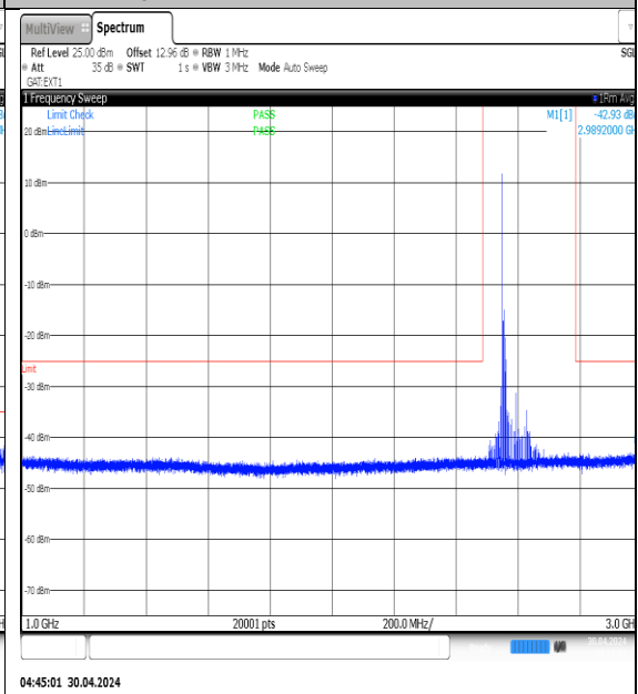
NTVN-N41-PC3-30-90-M-DFT-QPSK- Edge_1RB_Left-1000-3000-Ant1-PASS
