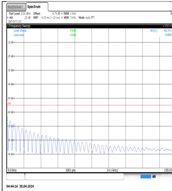
NTVN-N41-PC3-30-90-M-DFT-QPSK- Edge_1RB_Left-0.009-0.15-Ant1-PASS
