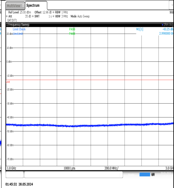
NTVN-N77-3450-3550-PC3-30-25-M-DFT-QPSK-Edge_1RB_Left-1000-3000-Ant1-PASS
