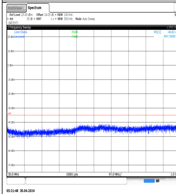
NTV-N41-PC3-30-100-H-DFT-QPSK- Edge_1RB_Left-30-1000-Ant1-PASS
