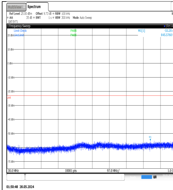
NTNV-N77-3450-3550-PC3-30-30-L-DFT-QPSK- Edge_1RB_Left-30-1000-Ant1-PASS
