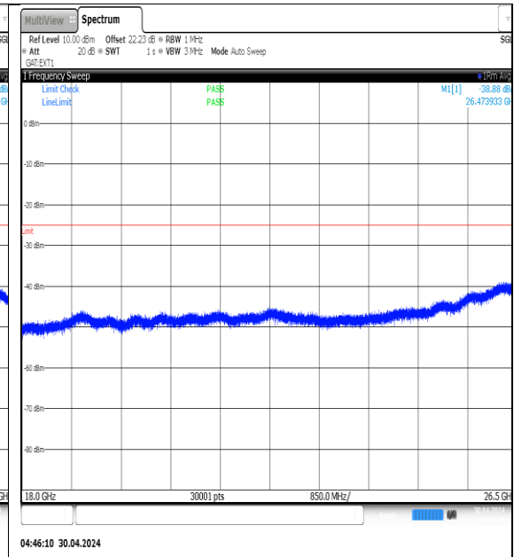
NTVN-N41-PC3-30-90-M-DFT-QPSK-Edge_1RB_Left-18000-26500-Ant1-PASS
