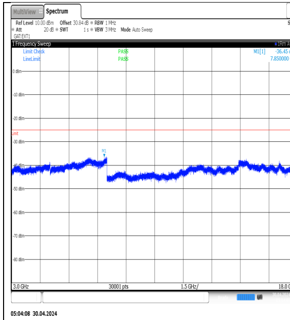
NTVN-N41-PC3-30-100-L-DFT-QPSK- Edge_1RB_Left-3000-18000-Ant1-PASS
