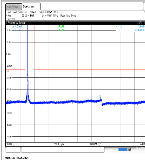
NTNV-N77-3450-3550-PC3-30-30-L-DFT-QPSK- Edge_1RB_Left-3000-6000-Ant1-PASS
