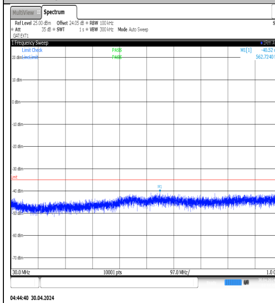
NTVN-N41-PC3-30-90-M-DFT-QPSK- Edge_1RB_Left-30-1000-Ant1-PASS
