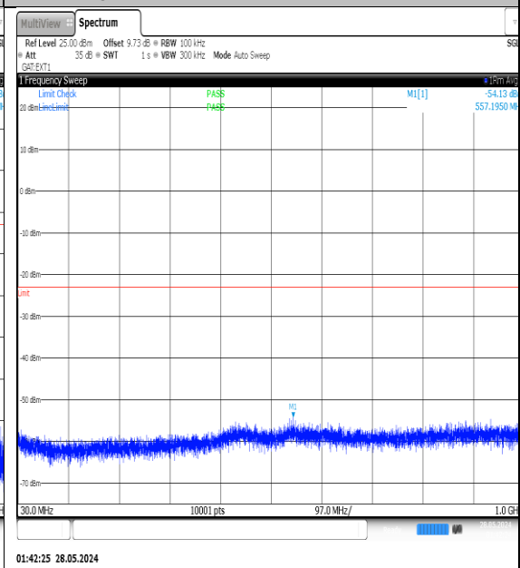
NTNV-N77-3450-3550-PC3-30-25-L-DFT-QPSK-Edge_1RB_Left-30-1000-Ant1-PASS
