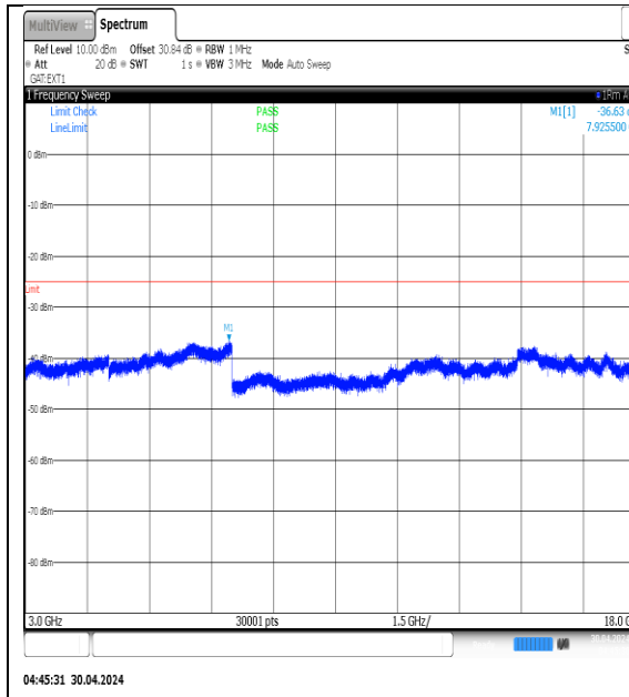
NTVN-N41-PC3-30-90-M-DFT-QPSK-Edge_1RB_Left-3000-18000-Ant1-PASS
