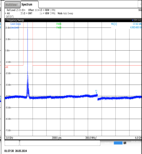
NTNV-N77-3450-3550-PC3-30-20-M-DFT-QPSK-Edge_1RB_Left-3000-6000-Ant1-PASS
