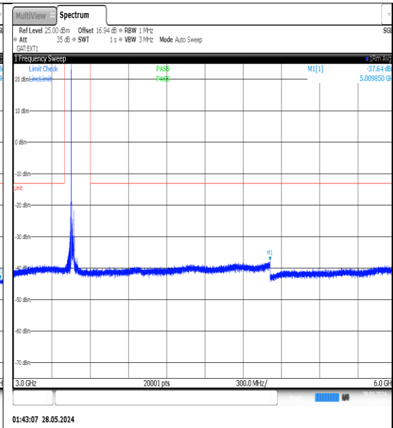
NTNV-N77-3450-3550-PC3-30-25-L-DFT-QPSK- Edge_1RB_Left-3000-6000-Ant1-PASS
