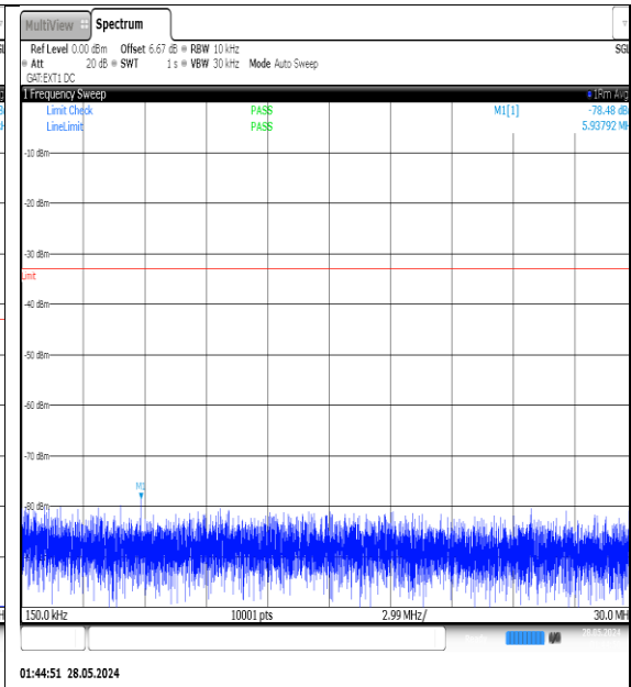
NTVN-N77-3450-3550-PC3-30-25-M-DFT-QPSK-Edge_1RB_Left-0.15-30-Ant1-PASS
