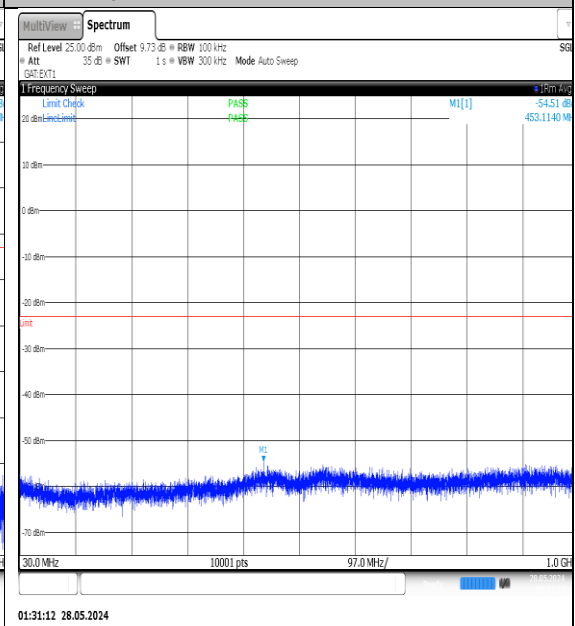
NTVN-N77-3450-3550-PC3-30-15-H-DFT-QPSK-Edge_1RB_Left-30-1000-Ant1-PASS
