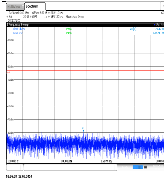
NTNV-N77-3450-3550-PC3-30-20-M-DFT-QPSK-Edge_1RB_Left-0.15-30-Ant1-PASS
