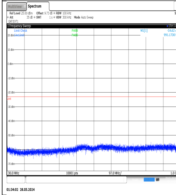
NTNV-N77-3450-3550-PC3-30-20-L-DFT-QPSK- Edge_1RB_Left-30-1000-Ant1-PASS
