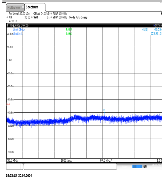
NTVN-N41-PC3-30-100-L-DFT-QPSK- Edge_1RB_Left-30-1000-Ant1-PASS
