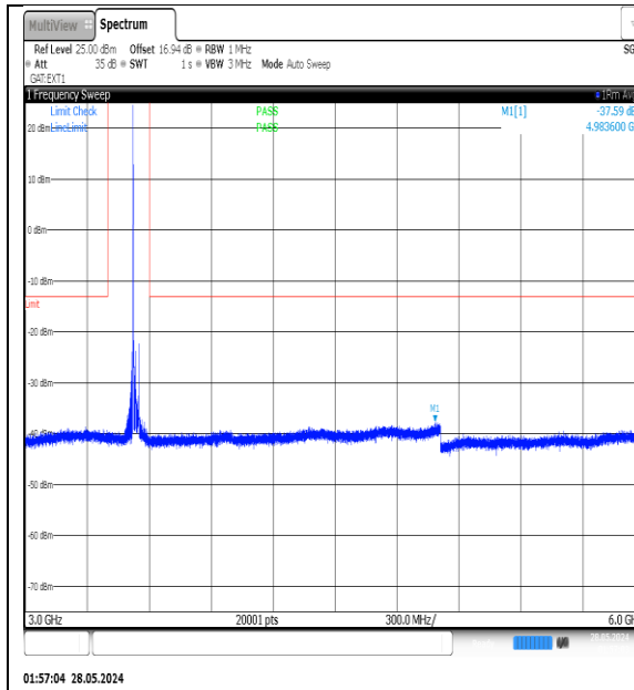
NTVN-N77-3450-3550-PC3-30-30-H-DFT-QPSK-Edge_1RB_Left-3000-6000-Ant1-PASS
