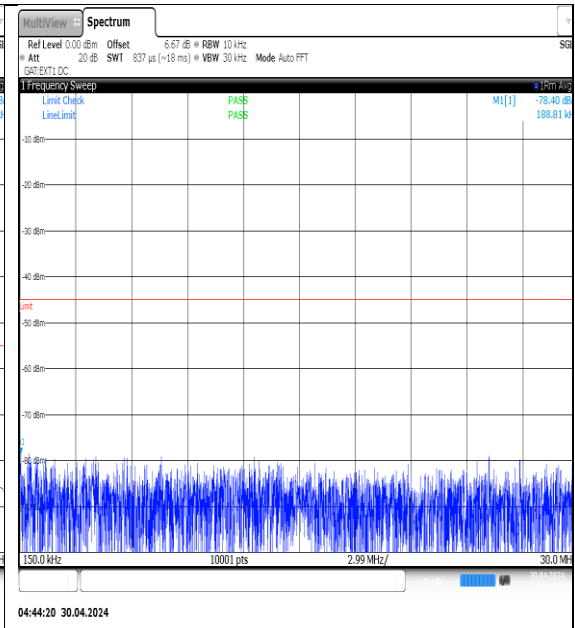
NTVN-N41-PC3-30-90-M-DFT-QPSK- Edge_1RB_Left-0.15-30-Ant1-PASS
