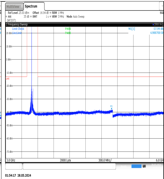
NTNV-N77-3450-3550-PC3-30-30-M-DFT-QPSK-Edge_1RB_Left-3000-6000-Ant1-PASS
