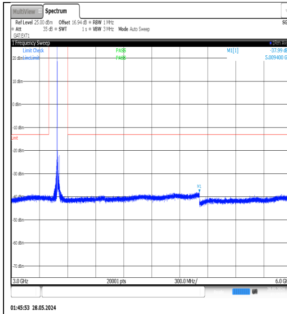
NTNV-N77-3450-3550-PC3-30-25-M-DFT-QPSK- Edge_1RB_Left-3000-6000-Ant1-PASS
