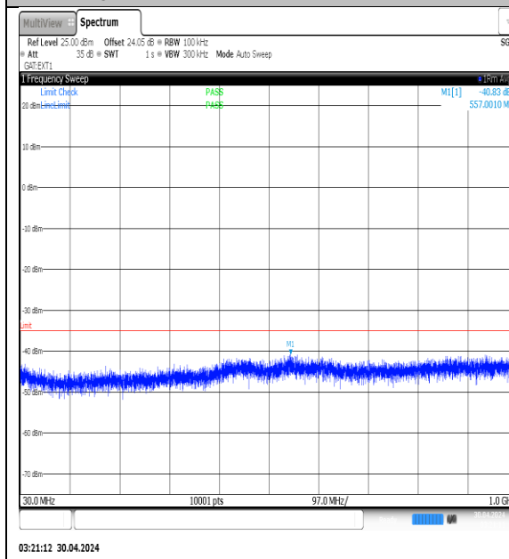
NTVN-N41-PC3-30-50-M-DFT-QPSK- Edge_1RB_Left-30-1000-Ant1-PASS
