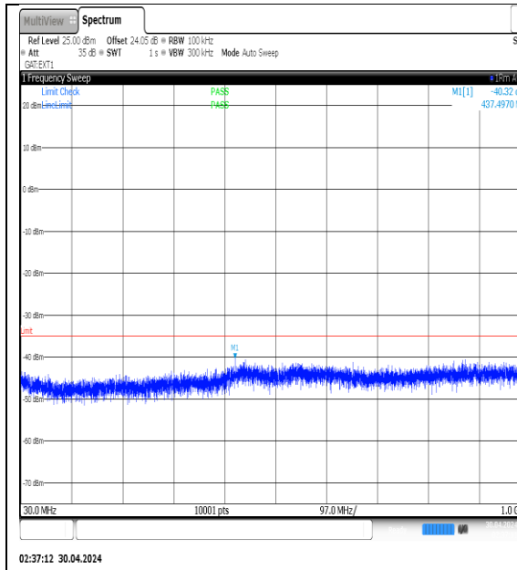
NTNV-N41-PC3-30-30-L-DFT-QPSK- Edge_1RB_Left-30-1000-Ant1-PASS
