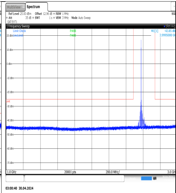
NTNV-N41-PC3-30-40-M-DFT-QPSK- Edge_1RB_Left-1000-3000-Ant1-PASS
