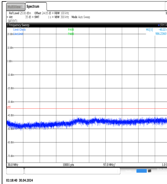
NTNV-N41-PC3-30-20-M-DFT-QPSK- Edge_1RB_Left-30-1000-Ant1-PASS
