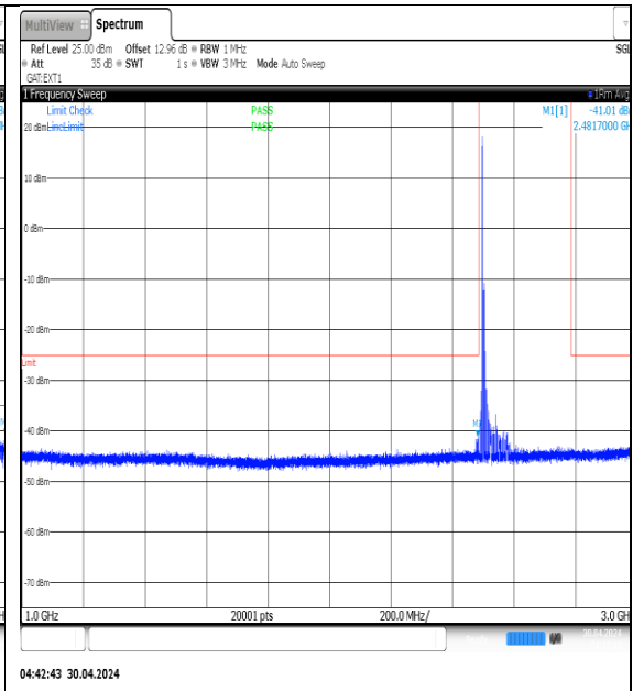
NTVN-N41-PC3-30-90-L-DFT-QPSK-Edge_1RB_Left-1000-3000-Ant1-PASS
