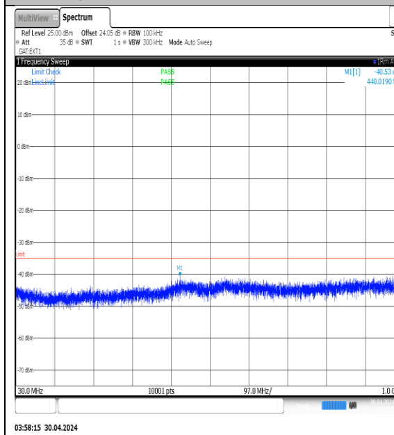
NTVN-N41-PC3-30-60-H-DFT-QPSK- Edge_1RB_Left-30-1000-Ant1-PASS
