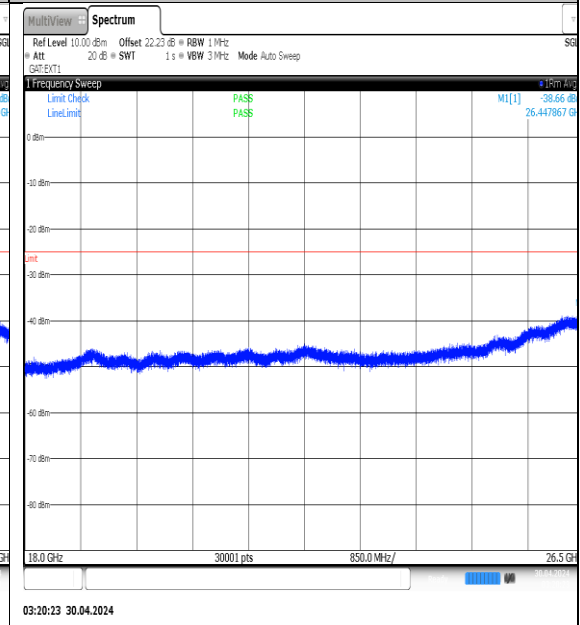
NTVN-N41-PC3-30-50-L-DFT-QPSK-Edge_1RB_Left-18000-26500-Ant1-PASS
