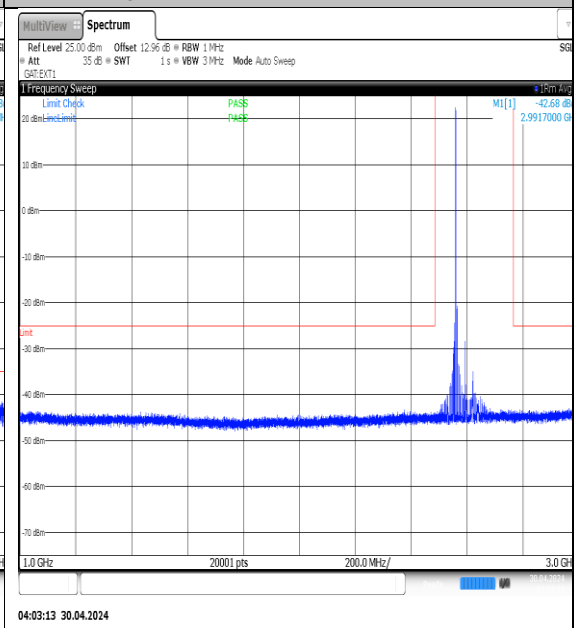
NTVN-N41-PC3-30-70-M-DFT-QPSK-Edge_1RB_Left-1000-3000-Ant1-PASS
