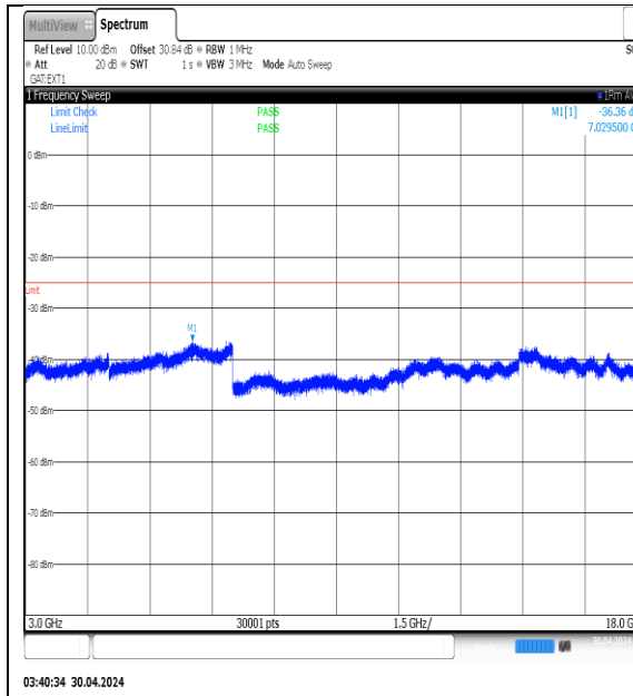
NTVN-N41-PC3-30-60-L-DFT-QPSK-Edge_1RB_Left-3000-18000-Ant1-PASS
