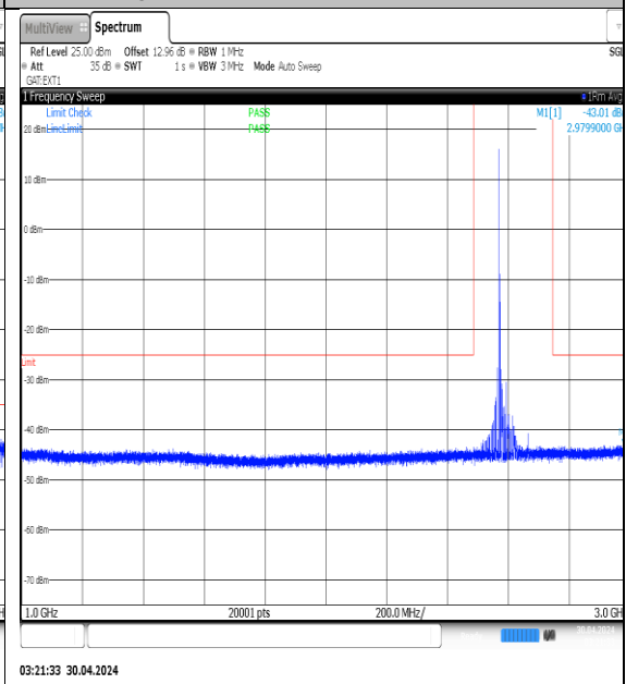
NTVN-N41-PC3-30-50-M-DFT-QPSK- Edge_1RB_Left-1000-3000-Ant1-PASS
