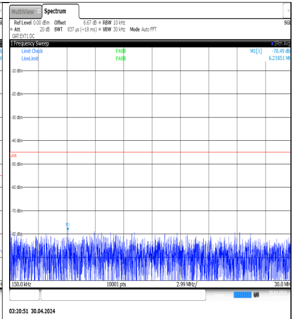
NTVN-N41-PC3-30-50-M-DFT-QPSK- Edge_1RB_Left-0.15-30-Ant1-PASS
