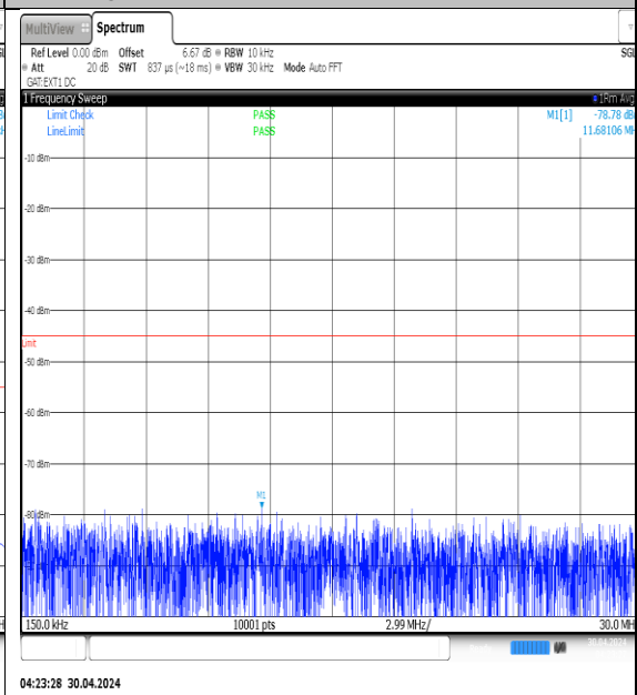
NTVN-N41-PC3-30-80-M-DFT-QPSK- Edge_1RB_Left-0.15-30-Ant1-PASS
