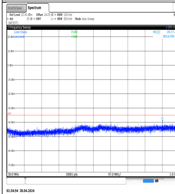
NTVN-N41-PC3-30-20-H-DFT-QPSK- Edge_1RB_Left-30-1000-Ant1-PASS
