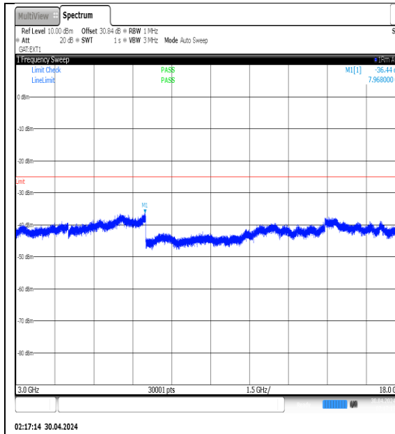
NTVN-N41-PC3-30-20-L-DFT-QPSK- Edge_1RB_Left-3000-18000-Ant1-PASS
