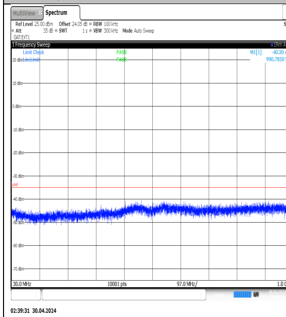
NTVN-N41-PC3-30-30-M-DFT-QPSK-Edge_1RB_Left-30-1000-Ant1-PASS
