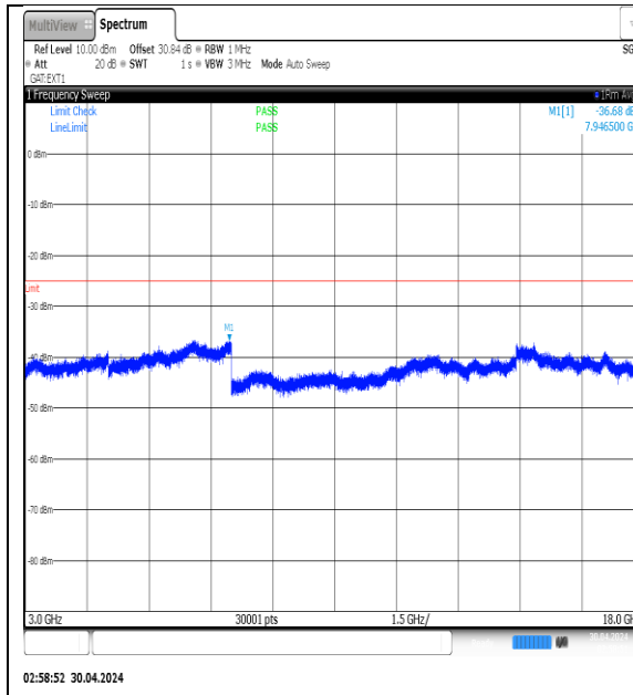
NTVN-N41-PC3-30-40-L-DFT-QPSK- Edge_1RB_Left-3000-18000-Ant1-PASS
