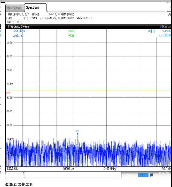
NTVN-N41-PC3-30-30-L-DFT-QPSK-Edge_1RB_Left-0.15-30-Ant1-PASS
