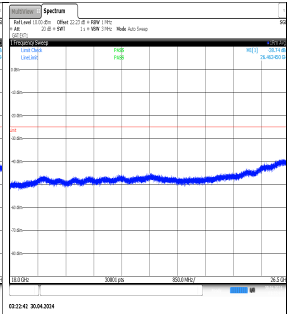
NTVN-N41-PC3-30-50-M-DFT-QPSK-Edge_1RB_Left-18000-26500-Ant1-PASS
