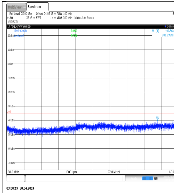
NTNV-N41-PC3-30-40-M-DFT-QPSK- Edge_1RB_Left-30-1000-Ant1-PASS
