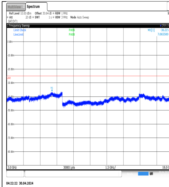
NTVN-N41-PC3-30-80-L-DFT-QPSK- Edge_1RB_Left-3000-18000-Ant1-PASS
