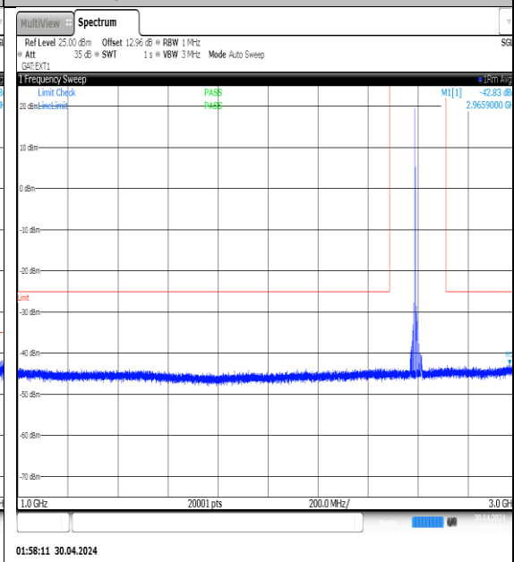
NTVN-N41-PC3-30-15-M-DFT-QPSK-Edge_1RB_Left-1000-3000-Ant1-PASS
