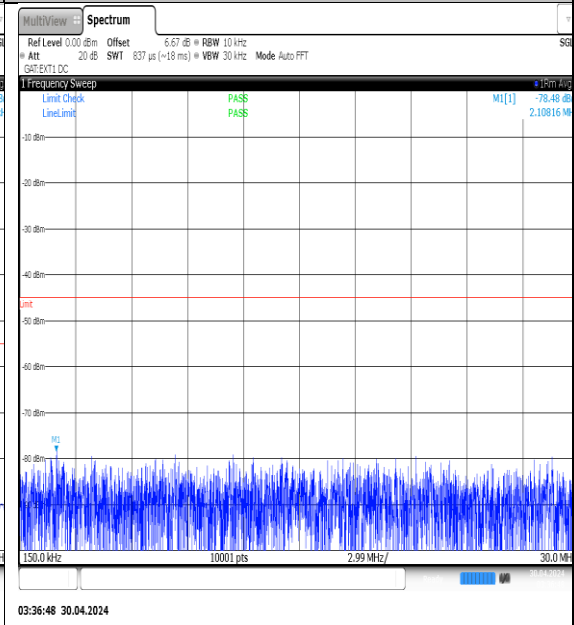
NTVN-N41-PC3-30-50-H-DFT-QPSK-Edge_1RB_Left-0.15-30-Ant1-PASS
