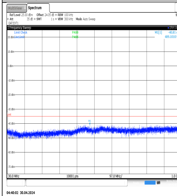
NTVN-N41-PC3-30-80-H-DFT-QPSK- Edge_1RB_Left-30-1000-Ant1-PASS
