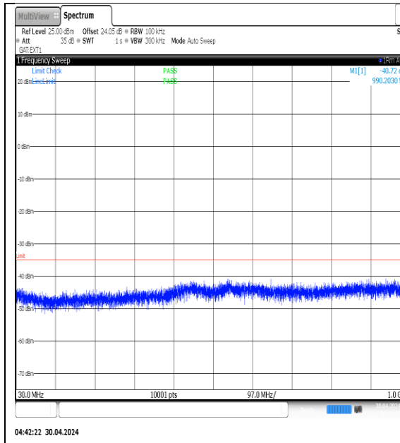
NTVN-N41-PC3-30-90-L-DFT-QPSK-Edge_1RB_Left-30-1000-Ant1-PASS
