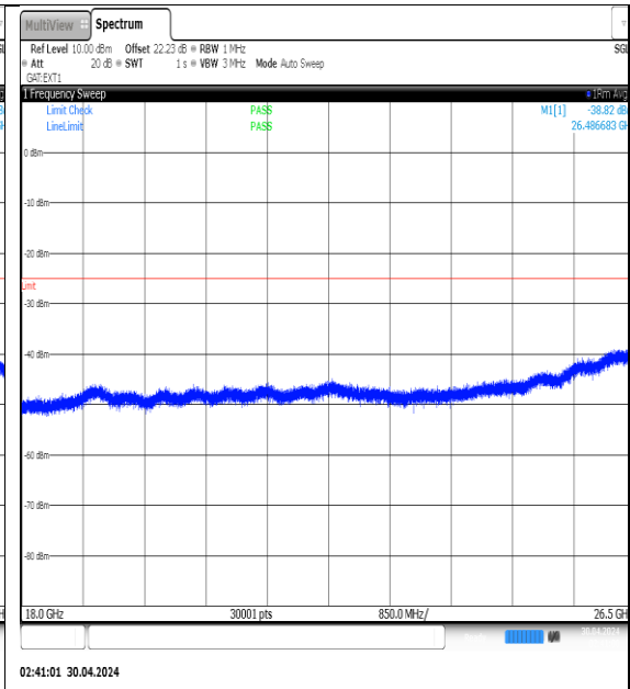
NTVN-N41-PC3-30-30-M-DFT-QPSK- Edge_1RB_Left-18000-26500-Ant1-PASS
