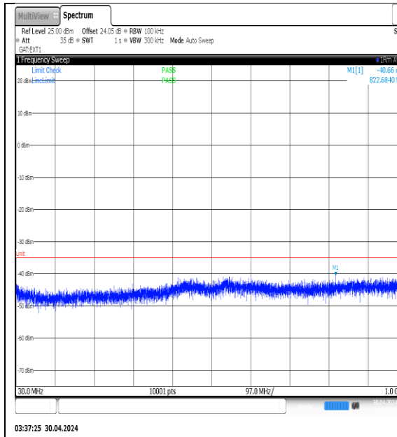
NTNV-N41-PC3-30-50-H-DFT-QPSK- Edge_1RB_Left-30-1000-Ant1-PASS
