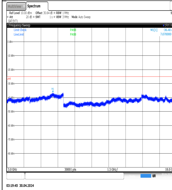
NTVN-N41-PC3-30-50-L-DFT-QPSK-Edge_1RB_Left-3000-18000-Ant1-PASS
