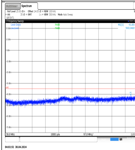
NTVN-N41-PC3-30-70-M-DFT-QPSK-Edge_1RB_Left-30-1000-Ant1-PASS
