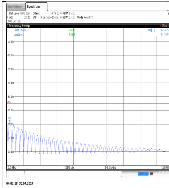
NTVN-N41-PC3-30-70-M-DFT-QPSK-Edge_1RB_Left-0.009-0.15-Ant1-PASS
