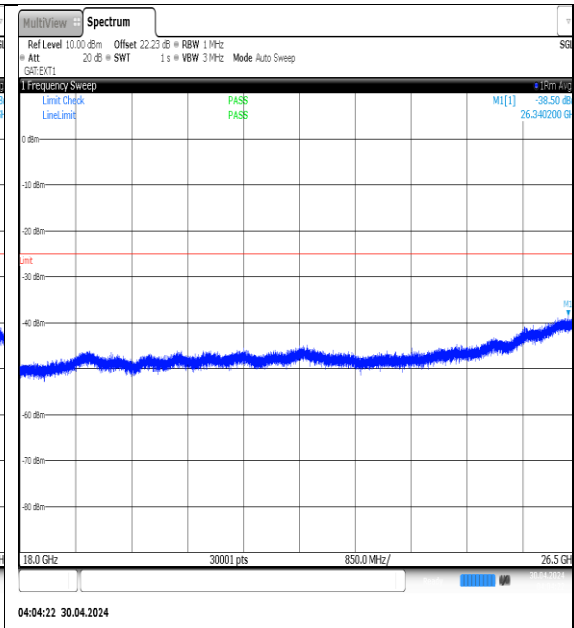
NTVN-N41-PC3-30-70-M-DFT-QPSK-Edge_1RB_Left-18000-26500-Ant1-PASS
