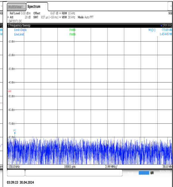
NTVN-N41-PC3-30-60-L-DFT-QPSK-Edge_1RB_Left-0.15-30-Ant1-PASS
