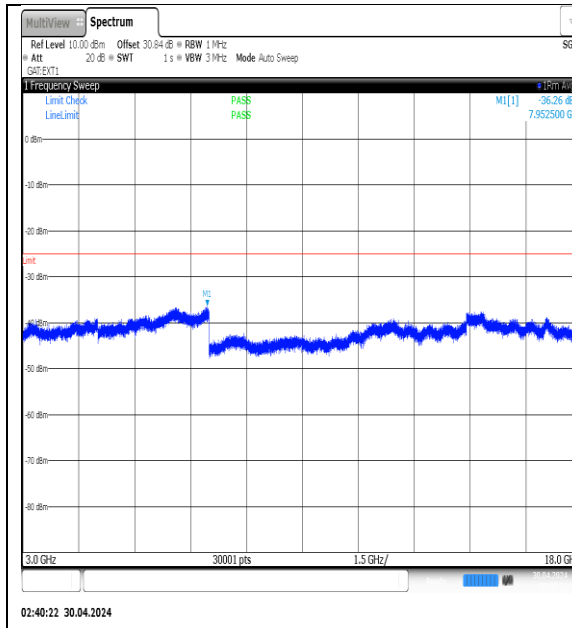
NTVN-N41-PC3-30-30-M-DFT-QPSK- Edge_1RB_Left-3000-18000-Ant1-PASS
