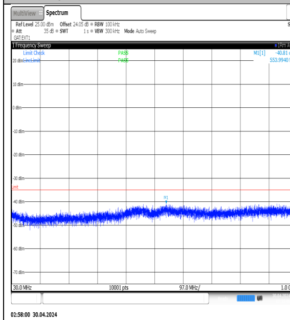
NTVN-N41-PC3-30-40-L-DFT-QPSK-Edge_1RB_Left-30-1000-Ant1-PASS
