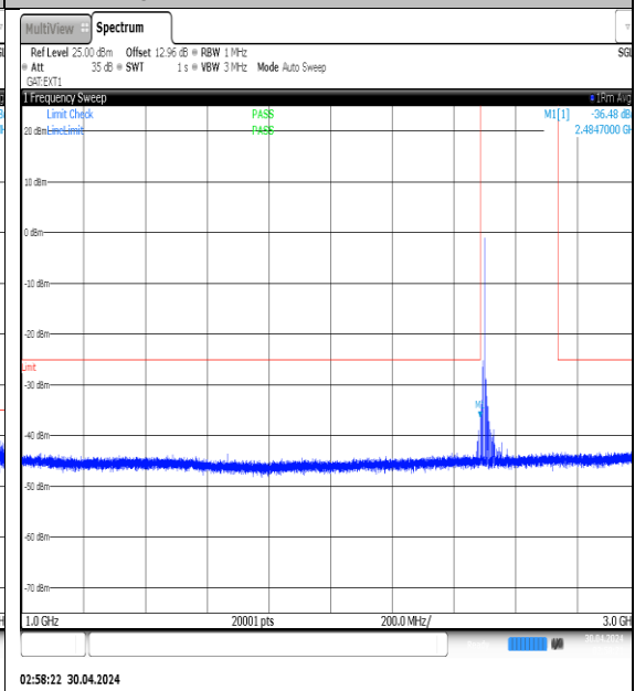
NTVN-N41-PC3-30-40-L-DFT-QPSK-Edge_1RB_Left-1000-3000-Ant1-PASS
