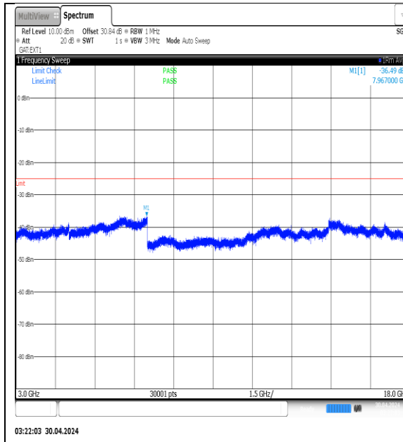
NTVN-N41-PC3-30-50-M-DFT-QPSK-Edge_1RB_Left-3000-18000-Ant1-PASS
