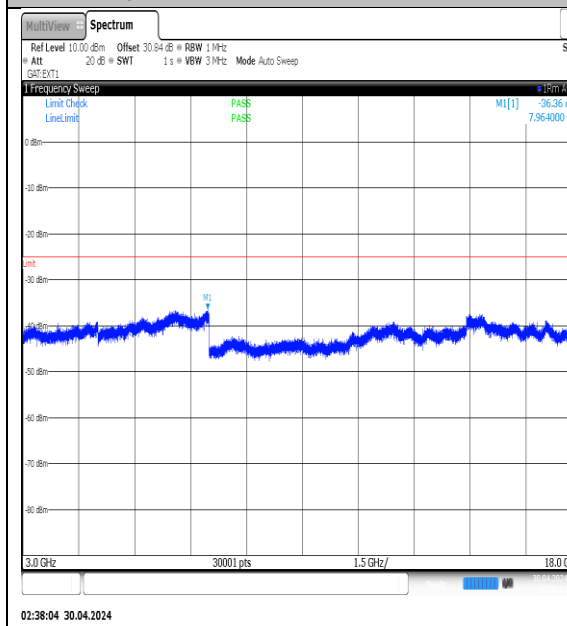
NTNV-N41-PC3-30-30-L-DFT-QPSK- Edge_1RB_Left-3000-18000-Ant1-PASS
