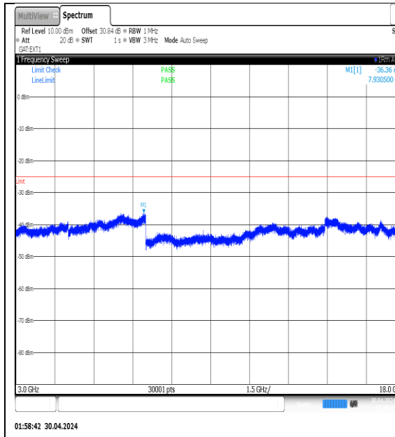
NTVN-N41-PC3-30-15-M-DFT-QPSK-Edge_1RB_Left-3000-18000-Ant1-PASS
