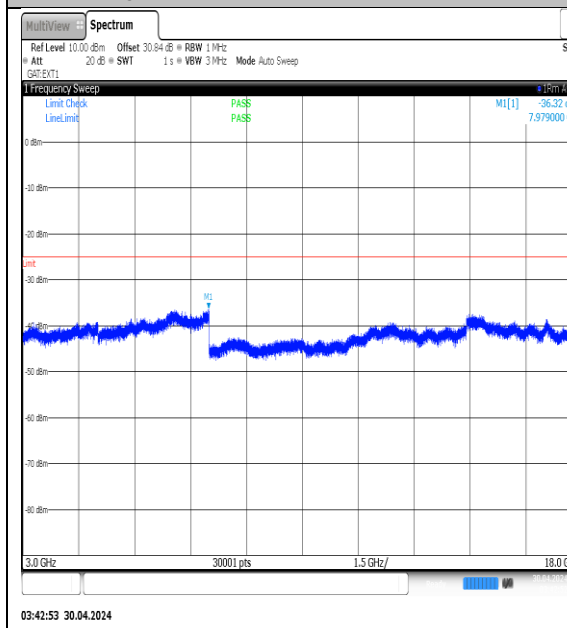
NTNV-N41-PC3-30-60-M-DFT-QPSK- Edge_1RB_Left-3000-18000-Ant1-PASS
