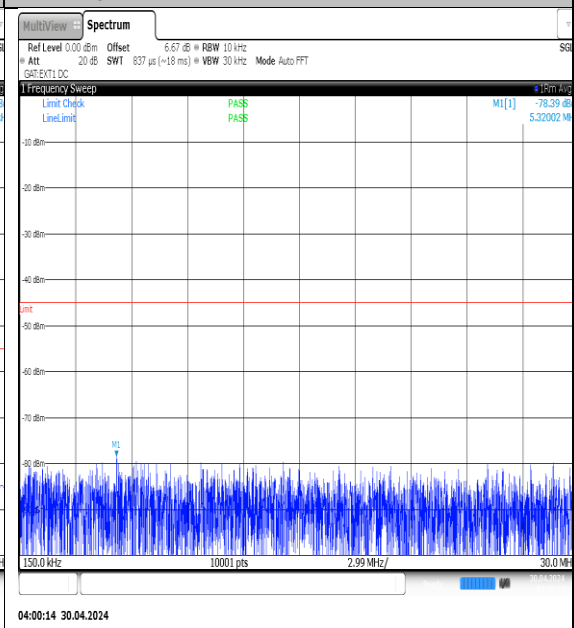
NTVN-N41-PC3-30-70-L-DFT-QPSK-Edge_1RB_Left-0.15-30-Ant1-PASS
