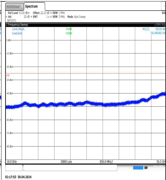
NTVN-N41-PC3-30-20-L-DFT-QPSK- Edge_1RB_Left-18000-26500-Ant1-PASS
