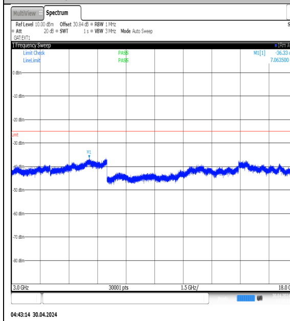
NTVN-N41-PC3-30-90-L-DFT-QPSK-Edge_1RB_Left-3000-18000-Ant1-PASS
