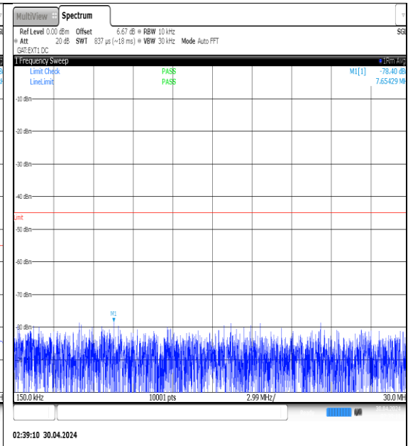
NTVN-N41-PC3-30-30-M-DFT-QPSK-Edge_1RB_Left-0.15-30-Ant1-PASS
