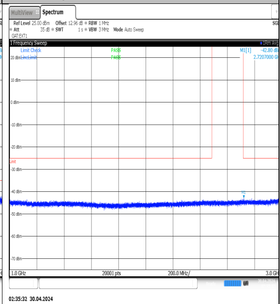
NTVN-N41-PC3-30-20-H-DFT-QPSK- Edge_1RB_Left-1000-3000-Ant1-PASS
