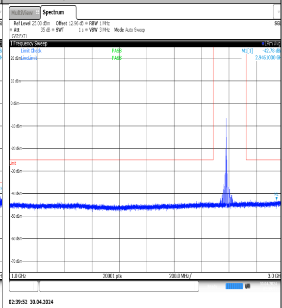
NTVN-N41-PC3-30-30-M-DFT-QPSK-Edge_1RB_Left-1000-3000-Ant1-PASS
