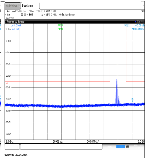
NTNV-N41-PC3-30-20-M-DFT-QPSK- Edge_1RB_Left-1000-3000-Ant1-PASS
