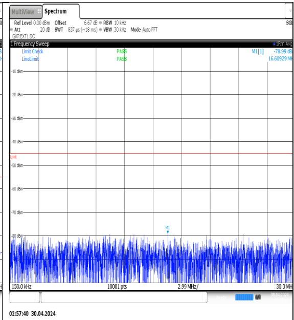
NTVN-N41-PC3-30-40-L-DFT-QPSK-Edge_1RB_Left-0.15-30-Ant1-PASS
