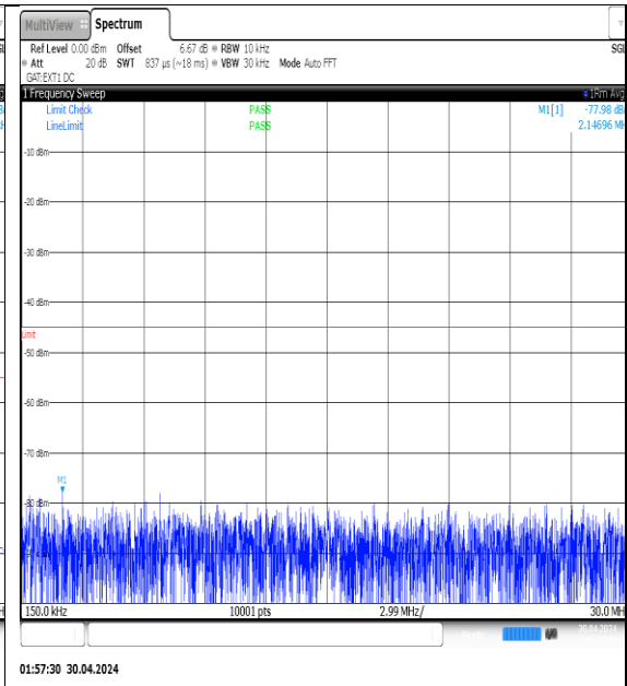
NTVN-N41-PC3-30-15-M-DFT-QPSK-Edge_1RB_Left-0.15-30-Ant1-PASS
