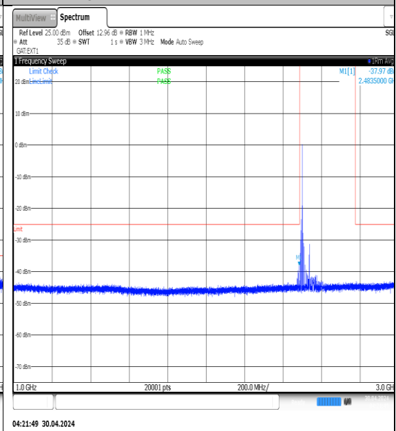
NTVN-N41-PC3-30-80-L-DFT-QPSK- Edge_1RB_Left-1000-3000-Ant1-PASS
