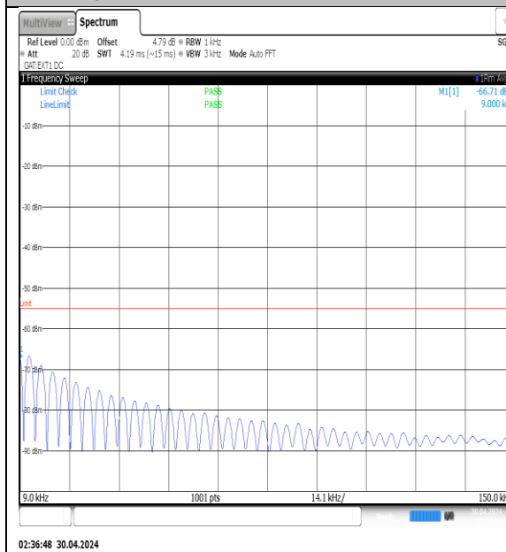
NTVN-N41-PC3-30-30-L-DFT-QPSK-Edge_1RB_Left-0.009-0.15-Ant1-PASS
