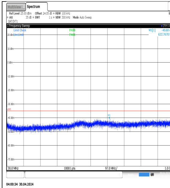
NTNV-N41-PC3-30-70-L-DFT-QPSK- Edge_1RB_Left-30-1000-Ant1-PASS
