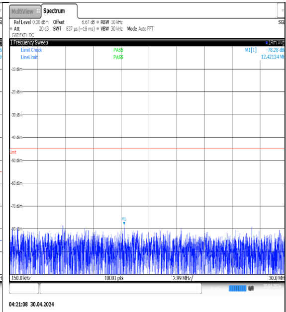
NTVN-N41-PC3-30-80-L-DFT-QPSK- Edge_1RB_Left-0.15-30-Ant1-PASS
