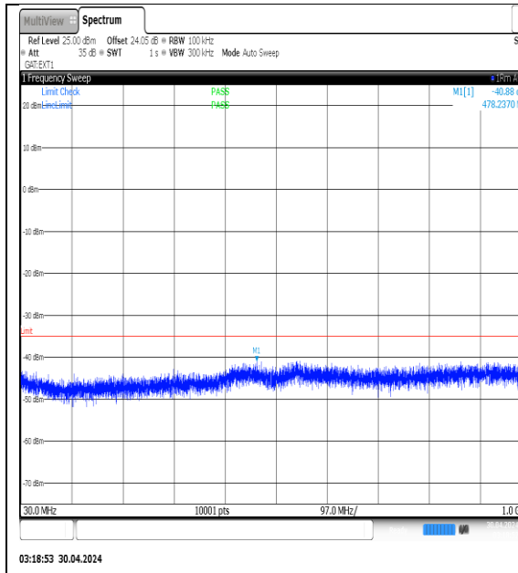
NTVN-N41-PC3-30-50-L-DFT-QPSK-Edge_1RB_Left-30-1000-Ant1-PASS
