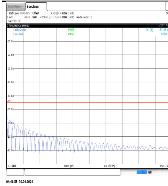
NTVN-N41-PC3-30-90-L-DFT-QPSK-Edge_1RB_Left-0.009-0.15-Ant1-PASS
