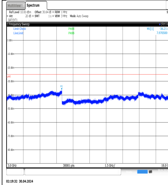
NTNV-N41-PC3-30-20-M-DFT-QPSK- Edge_1RB_Left-3000-18000-Ant1-PASS
