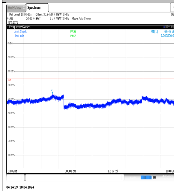
NTNV-N41-PC3-30-80-M-DFT-QPSK- Edge_1RB_Left-3000-18000-Ant1-PASS
