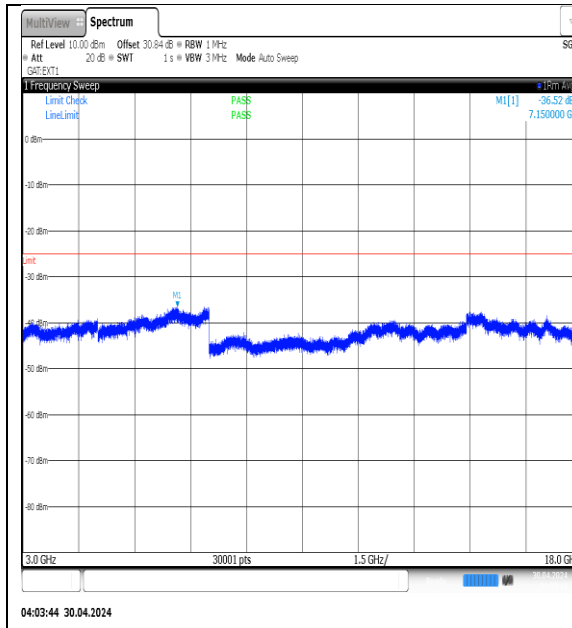
NTVN-N41-PC3-30-70-M-DFT-QPSK-Edge_1RB_Left-3000-18000-Ant1-PASS
