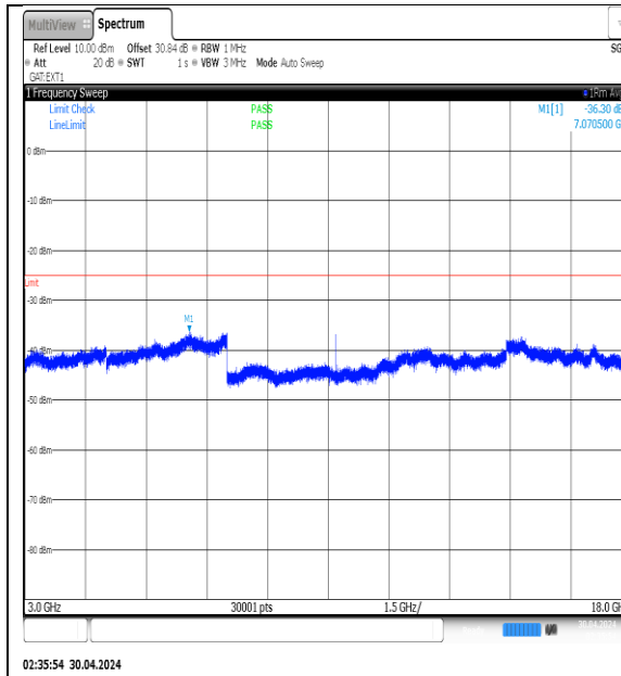
NTVN-N41-PC3-30-20-H-DFT-QPSK-Edge_1RB_Left-3000-18000-Ant1-PASS
