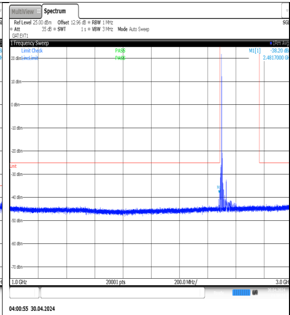
NTNV-N41-PC3-30-70-L-DFT-QPSK- Edge_1RB_Left-1000-3000-Ant1-PASS
