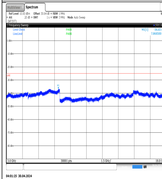
NTNV-N41-PC3-30-70-L-DFT-QPSK- Edge_1RB_Left-3000-18000-Ant1-PASS
