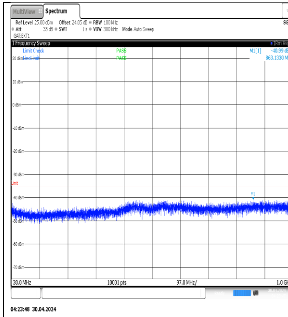
NTNV-N41-PC3-30-80-M-DFT-QPSK- Edge_1RB_Left-30-1000-Ant1-PASS
