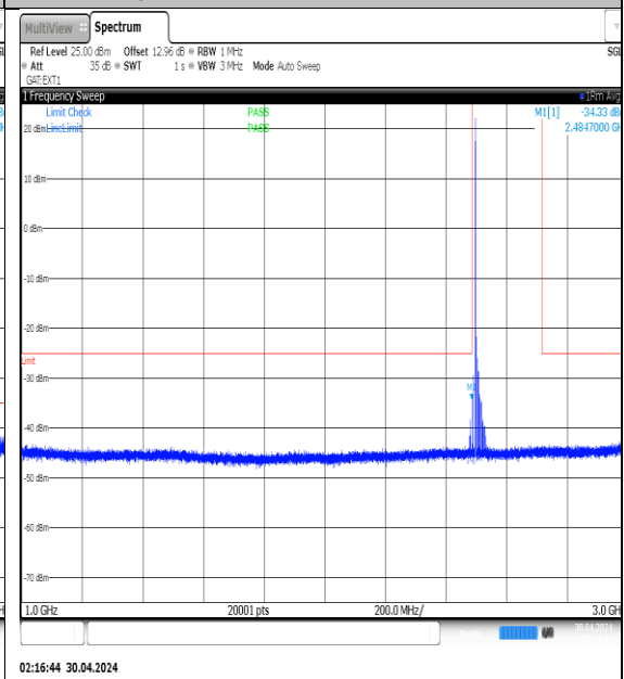
NTVN-N41-PC3-30-20-L-DFT-QPSK-Edge_1RB_Left-1000-3000-Ant1-PASS
