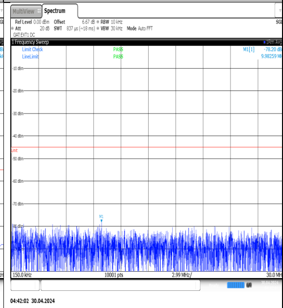
NTVN-N41-PC3-30-90-L-DFT-QPSK-Edge_1RB_Left-0.15-30-Ant1-PASS
