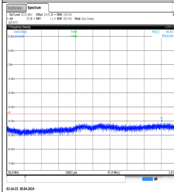
NTVN-N41-PC3-30-20-L-DFT-QPSK-Edge_1RB_Left-30-1000-Ant1-PASS
