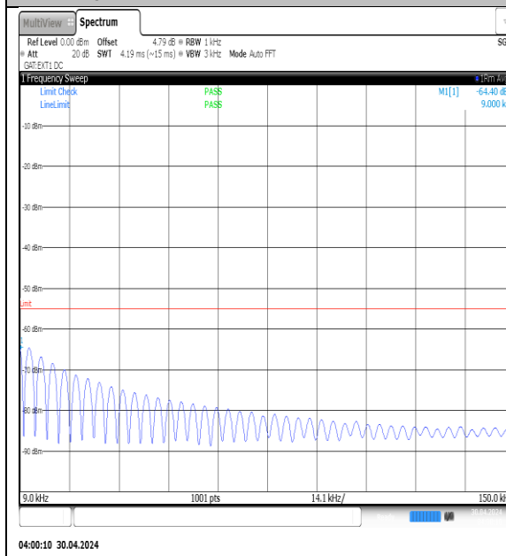
NTVN-N41-PC3-30-70-L-DFT-QPSK-Edge_1RB_Left-0.009-0.15-Ant1-PASS
