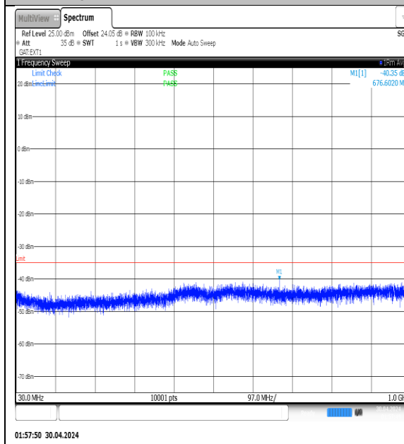
NTVN-N41-PC3-30-15-M-DFT-QPSK-Edge_1RB_Left-30-1000-Ant1-PASS
