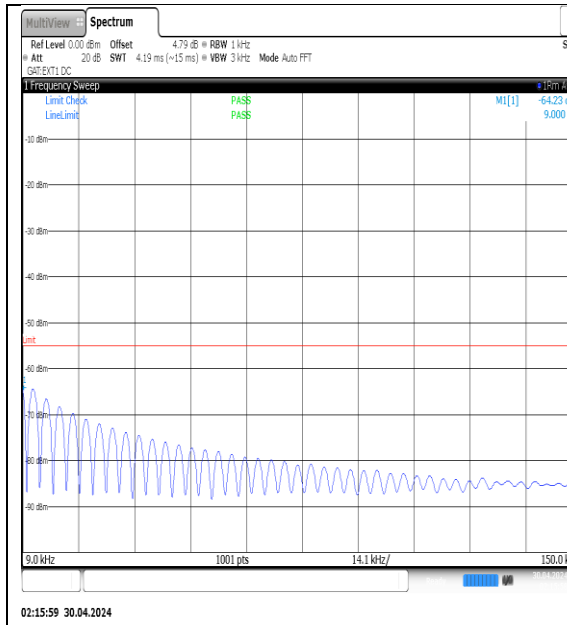
NTVN-N41-PC3-30-20-L-DFT-QPSK-Edge_1RB_Left-0.009-0.15-Ant1-PASS
