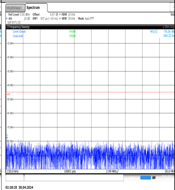
NTVN-N41-PC3-30-20-M-DFT-QPSK- Edge_1RB_Left-0.15-30-Ant1-PASS
