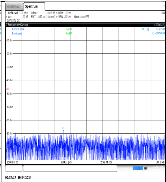
NTVN-N41-PC3-30-20-H-DFT-QPSK- Edge_1RB_Left-0.15-30-Ant1-PASS
