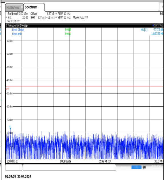
NTVN-N41-PC3-30-40-M-DFT-QPSK- Edge_1RB_Left-0.15-30-Ant1-PASS
