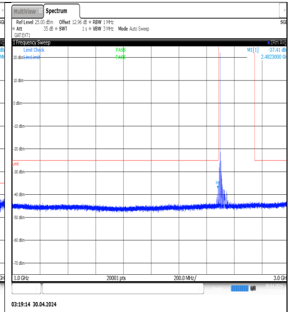
NTVN-N41-PC3-30-50-L-DFT-QPSK-Edge_1RB_Left-1000-3000-Ant1-PASS
