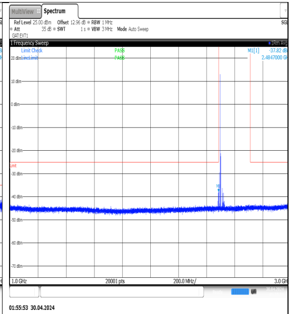
NTVN-N41-PC3-30-15-L-DFT-QPSK-Edge_1RB_Left-1000-3000-Ant1-PASS
