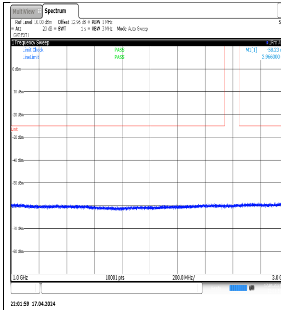
NTVN-N38-PC3-30-20-L-DFT-QPSK-Edge_1RB_Left-1000-3000-Ant1-PASS
