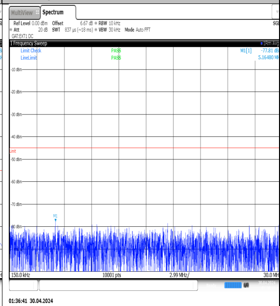
NTVN-N41-PC3-30-10-M-DFT-QPSK-Edge_1RB_Left-0.15-30-Ant1-PASS
