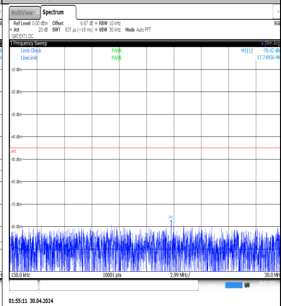
NTVN-N41-PC3-30-15-L-DFT-QPSK-Edge_1RB_Left-0.15-30-Ant1-PASS
