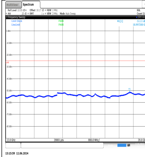
NTNV-N7-PC3-15-40-L-DFT-QPSK-Edge_1RB_Left-12000-20000-Ant1-PASS
