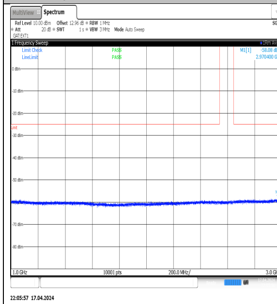
NTVN-N38-PC3-30-20-M-DFT-QPSK- Edge_1RB_Left-1000-3000-Ant1-PASS
