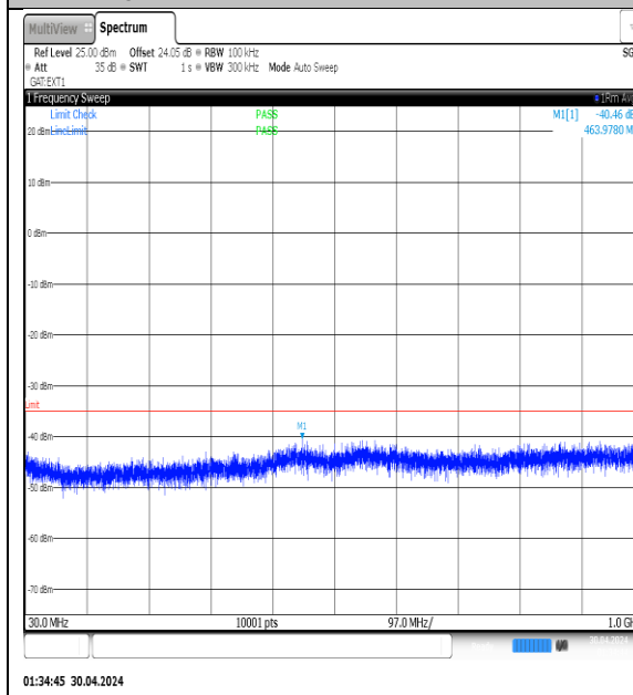
NTVN-N41-PC3-30-10-L-DFT-QPSK-Edge_1RB_Left-30-1000-Ant1-PASS
