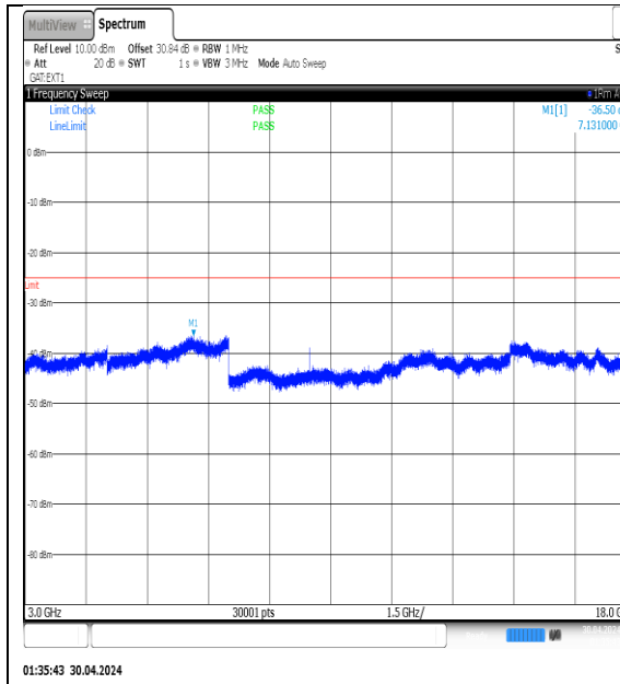
NTVN-N41-PC3-30-10-L-DFT-QPSK-Edge_1RB_Left-3000-18000-Ant1-PASS
