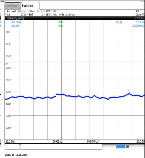
NTNV-N7-PC3-15-40-M-DFT-QPSK-Edge_1RB_Left-12000-20000-Ant1-PASS
