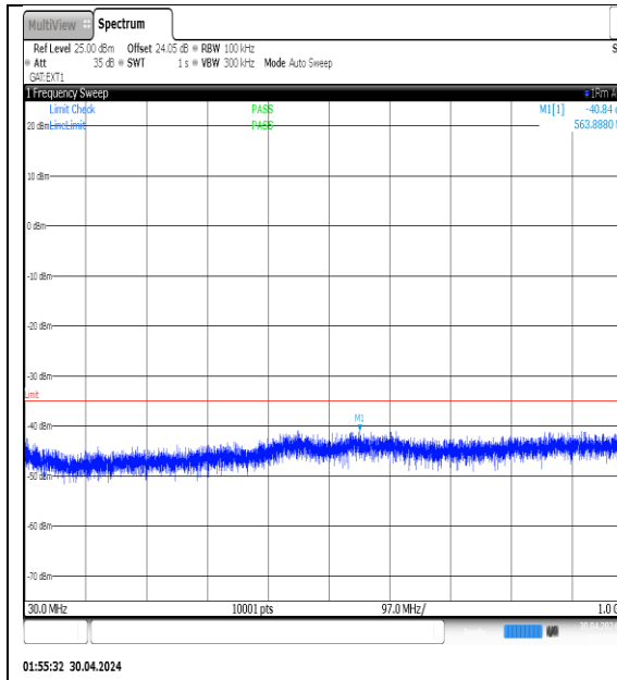
NTVN-N41-PC3-30-15-L-DFT-QPSK-Edge_1RB_Left-30-1000-Ant1-PASS
