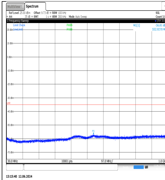
NTNV-N7-PC3-15-40-L-DFT-QPSK-Edge_1RB_Left-30-1000-Ant1-PASS
