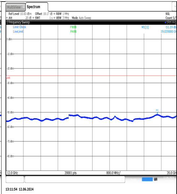
NTNV-N7-PC3-15-25-M-DFT-QPSK-Edge_1RB_Left-12000-20000-Ant1-PASS
