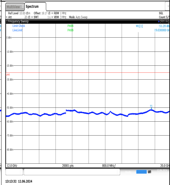
NTNV-N7-PC3-15-30-L-DFT-QPSK- Edge_1RB_Left-12000-20000-Ant1-PASS
