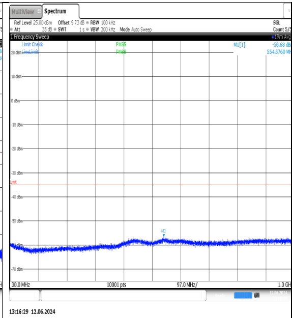
NTNV-N7-PC3-15-40-M-DFT-QPSK-Edge_1RB_Left-30-1000-Ant1-PASS
