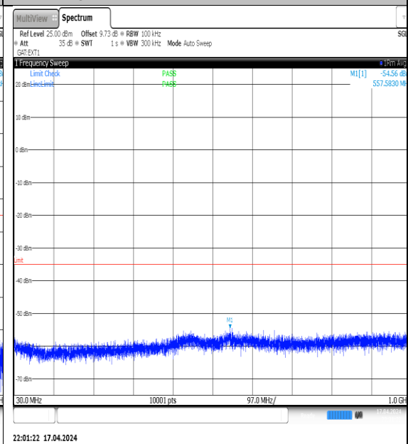
NTVN-N38-PC3-30-20-L-DFT-QPSK-Edge_1RB_Left-30-1000-Ant1-PASS
