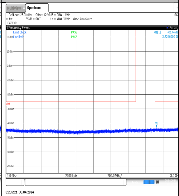
NTVN-N41-PC3-30-10-L-DFT-QPSK-Edge_1RB_Left-1000-3000-Ant1-PASS
