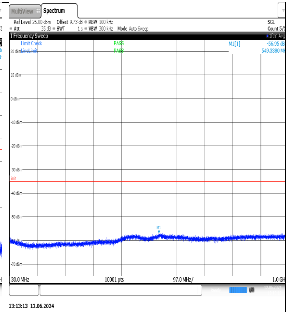
NTNV-N7-PC3-15-30-L-DFT-QPSK- Edge_1RB_Left-30-1000-Ant1-PASS
