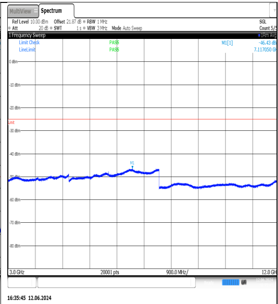
NTNV-N7-PC3-15-40-L-DFT-QPSK-Edge_1RB_Left-3000-12000-Ant1-PASS
