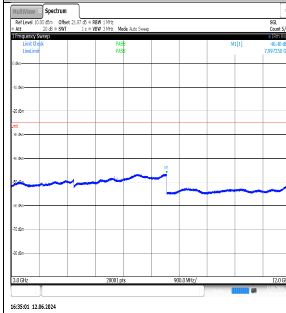
NTNV-N7-PC3-15-30-L-DFT-QPSK- Edge_1RB_Left-3000-12000-Ant1-PASS
