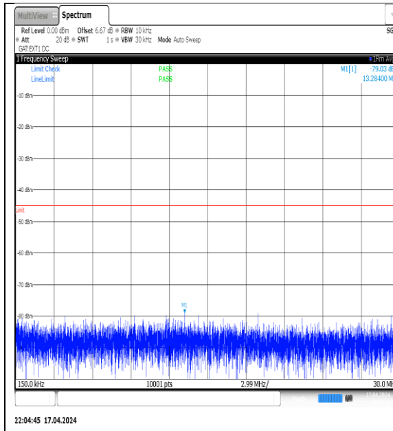
NTVN-N38-PC3-30-20-M-DFT-QPSK- Edge_1RB_Left-0.15-30-Ant1-PASS
