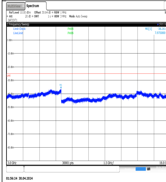
NTVN-N41-PC3-30-15-L-DFT-QPSK-Edge_1RB_Left-3000-18000-Ant1-PASS
