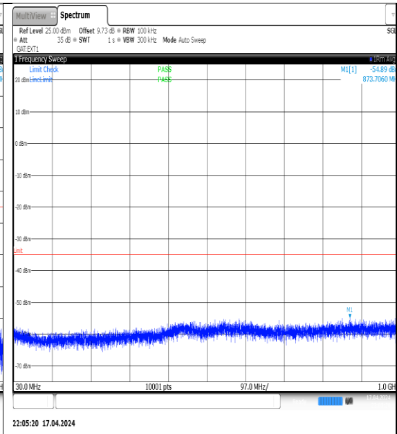
NTVN-N38-PC3-30-20-M-DFT-QPSK- Edge_1RB_Left-30-1000-Ant1-PASS
