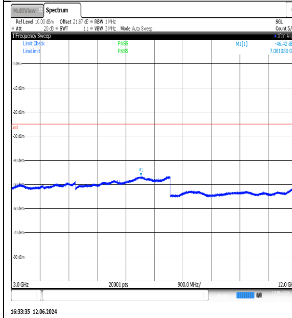
NTNV-N7-PC3-15-20-L-DFT-QPSK-Edge_1RB_Left-3000-12000-Ant1-PASS
