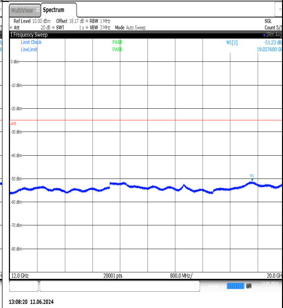
NTNV-N7-PC3-15-20-L-DFT-QPSK-Edge_1RB_Left-12000-20000-Ant1-PASS
