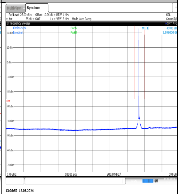
NTVN-N7-PC3-15-20-M-DFT-QPSK-Edge_1RB_Left-1000-3000-Ant1-PASS
