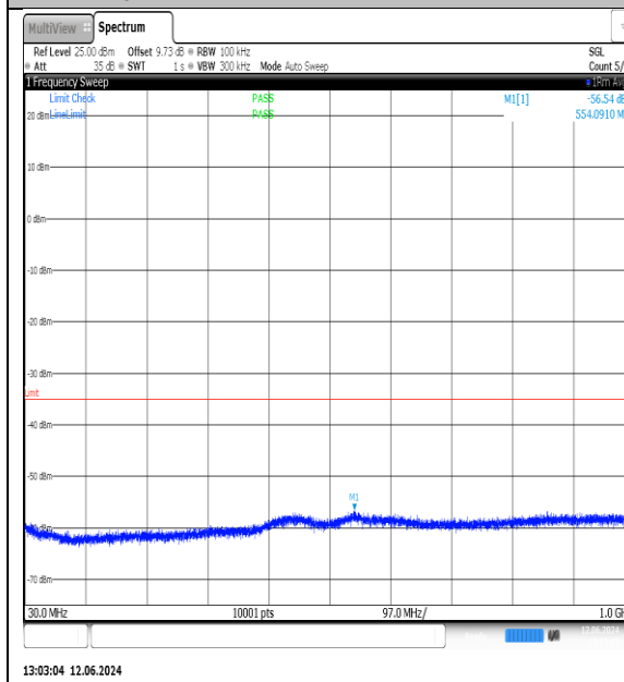
NTVN-N7-PC3-15-10-M-DFT-QPSK-Edge_1RB_Left-30-1000-Ant1-PASS
