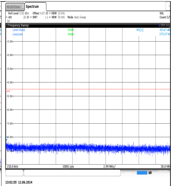
NTVN-N7-PC3-15-10-M-DFT-QPSK-Edge_1RB_Left-0.15-30-Ant1-PASS
