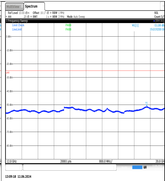
NTNV-N7-PC3-15-20-M-DFT-QPSK-Edge_1RB_Left-12000-20000-Ant1-PASS
