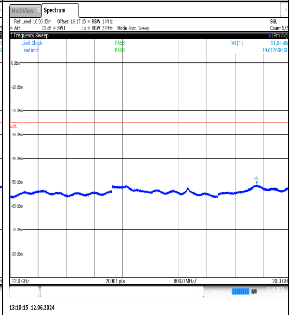
NTNV-N7-PC3-15-20-H-DFT-QPSK-Edge_1RB_Left-12000-20000-Ant1-PASS
