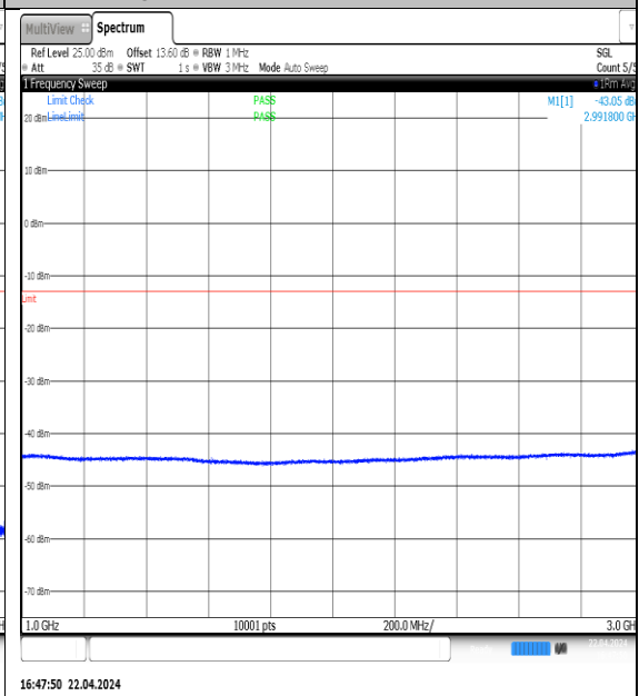
NTNV-N5-PC3-15-20-M-DFT-QPSK- Edge_1RB_Left-1000-3000-Ant1-PASS
