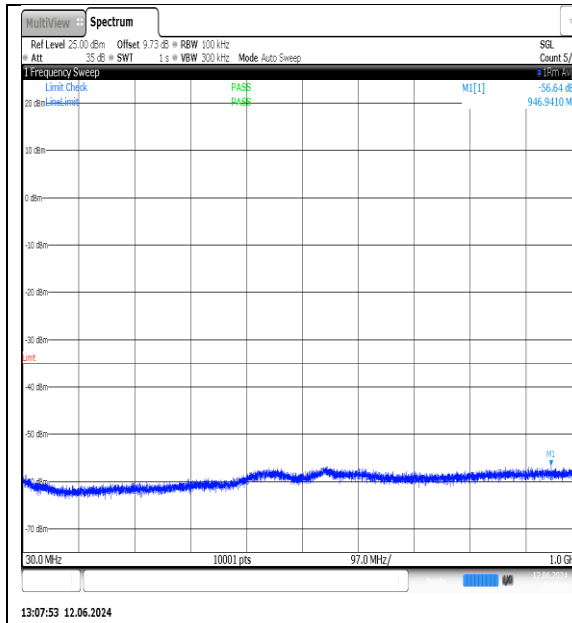
NTNV-N7-PC3-15-20-L-DFT-QPSK-Edge_1RB_Left-30-1000-Ant1-PASS
