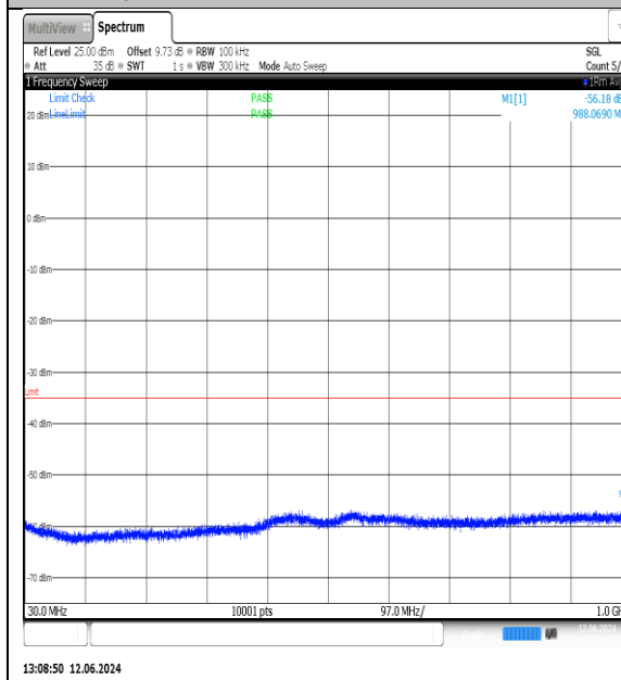
NTVN-N7-PC3-15-20-M-DFT-QPSK-Edge_1RB_Left-30-1000-Ant1-PASS
