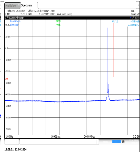
NTNV-N7-PC3-15-20-L-DFT-QPSK-Edge_1RB_Left-1000-3000-Ant1-PASS
