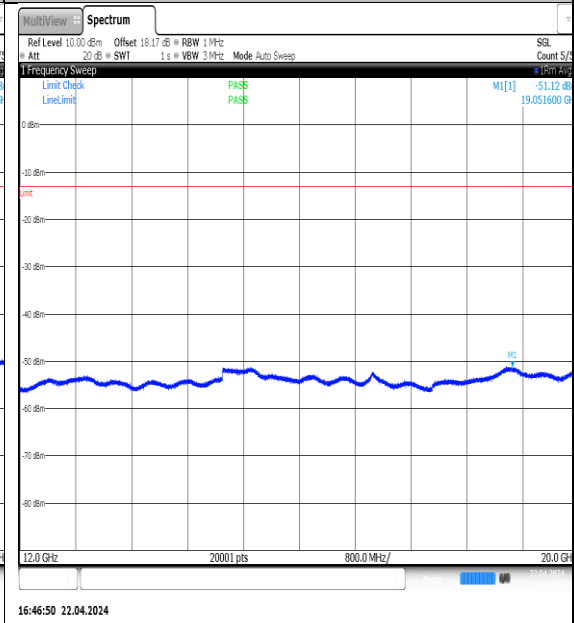
NTNV-N5-PC3-15-20-L-DFT-QPSK-Edge_1RB_Left-12000-20000-Ant1-PASS
