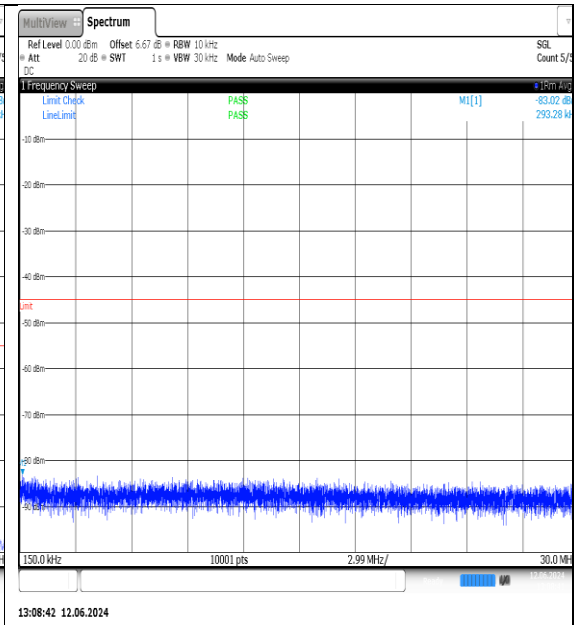
NTVN-N7-PC3-15-20-M-DFT-QPSK-Edge_1RB_Left-0.15-30-Ant1-PASS
