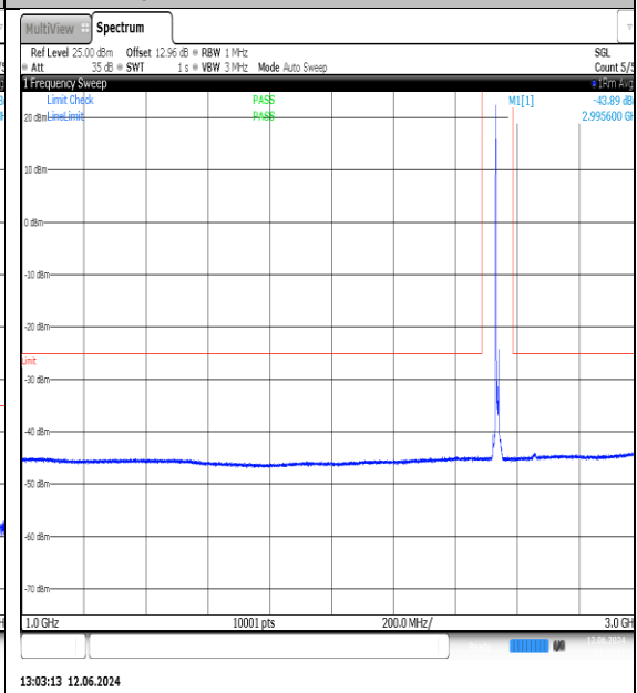
NTVN-N7-PC3-15-10-M-DFT-QPSK-Edge_1RB_Left-1000-3000-Ant1-PASS
