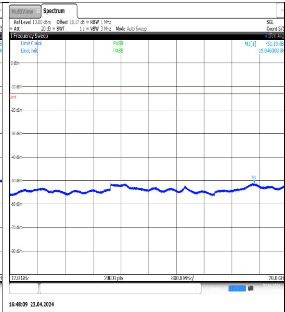
NTNV-N5-PC3-15-20-M-DFT-QPSK-Edge_1RB_Left-12000-20000-Ant1-PASS
