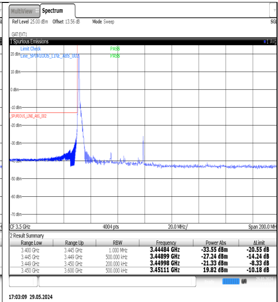
NTNV-N77-3450-3550-PC3-30-50-L-DFT-QPSK-Edge_1RB_Left-Ant1-PASS
