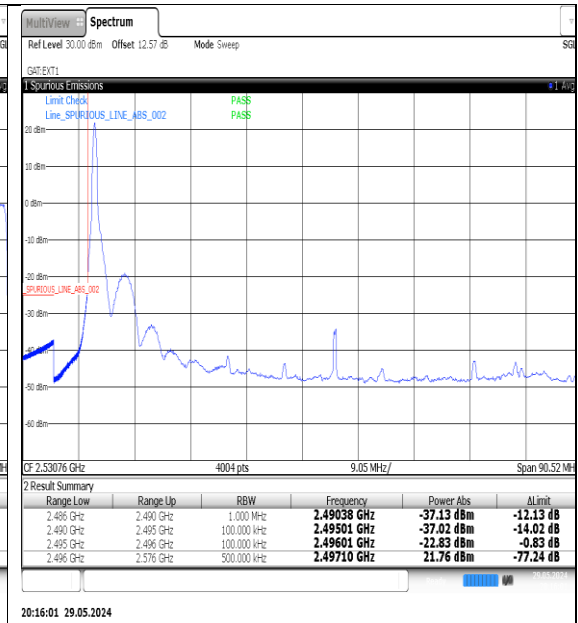
NTNV-N41-PC3-30-80-L-DFT-QPSK-Edge_1RB_Left-Ant1-PASS
