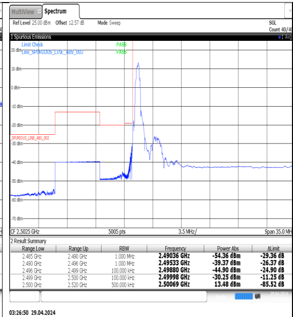
NTNV-N7-PC3-15-40-L-DFT-QPSK-Edge_1RB_Left-Ant1-PASS
