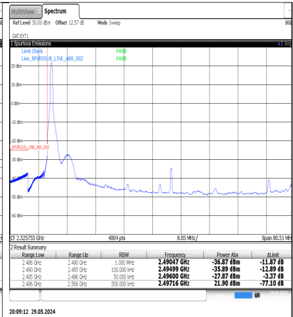
NTNV-N41-PC3-30-70-L-DFT-QPSK-Edge_1RB_Left-Ant1-PASS
