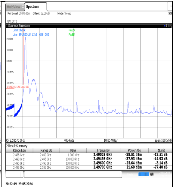
NTNV-N41-PC3-30-90-L-DFT-QPSK-Edge_1RB_Left-Ant1-PASS
