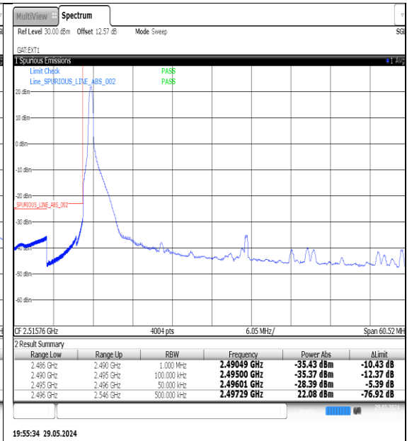
NTNV-N41-PC3-30-50-L-DFT-QPSK-Edge_1RB_Left-Ant1-PASS
