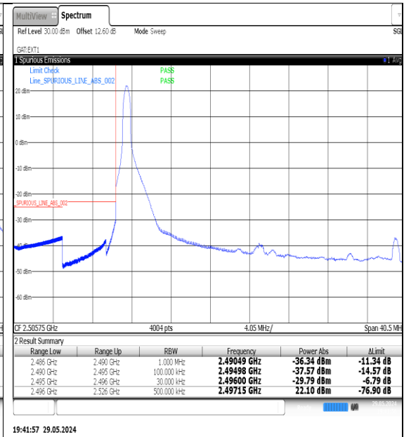
NTNV-N41-PC3-30-30-L-DFT-QPSK-Edge_1RB_Left-Ant1-PASS
