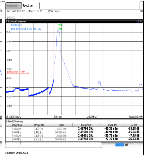
NTNV-N41-PC3-30-20-L-DFT-QPSK-Edge_1RB_Left-Ant1-PASS
