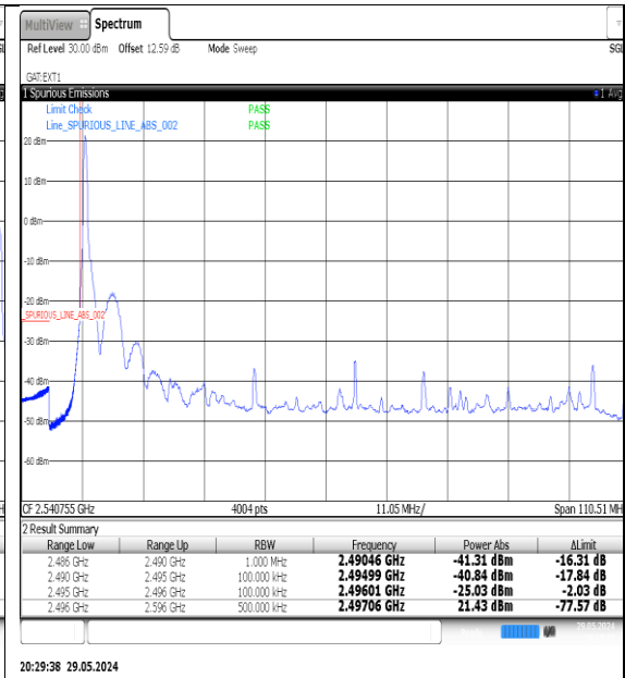
NTVN-N41-PC3-30-100-L-DFT-QPSK-Edge_1RB_Left-Ant1-PASS
