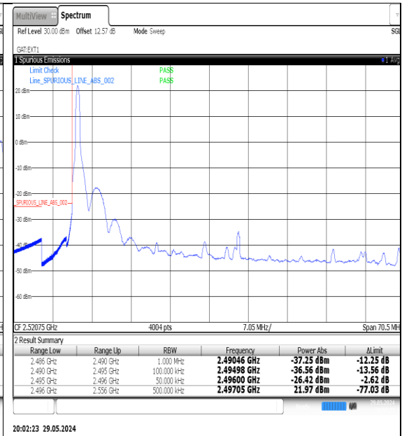
NTNV-N41-PC3-30-60-L-DFT-QPSK-Edge_1RB_Left-Ant1-PASS
