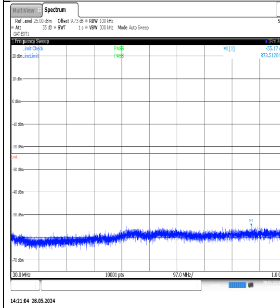
NTNV-N77-3700-3980-PC3-30-20-L-DFT-QPSK- Edge_1RB_Left-30-1000-Ant1-PASS
