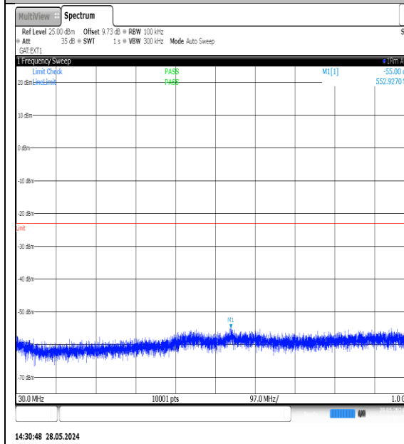
NTVN-N77-3700-3980-PC3-30-25-M-DFT-QPSK-Edge_1RB_Left-30-1000-Ant1-PASS
