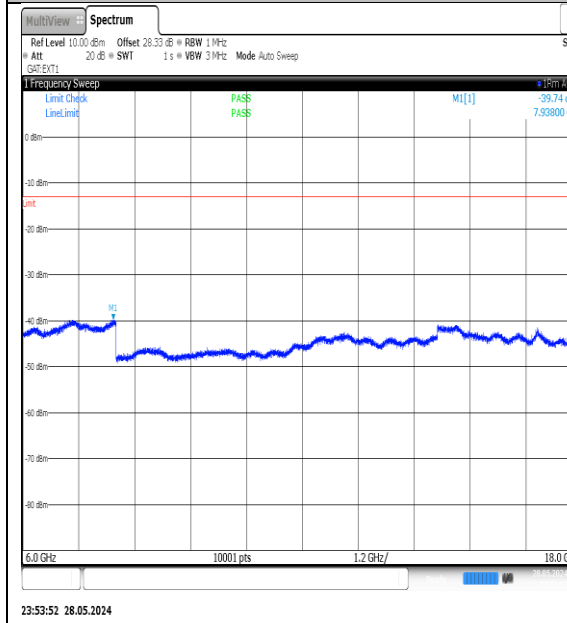
NTNV-N78-3700-3800-PC3-30-90-M-DFT-QPSK- Edge_1RB_Left-6000-18000-Ant1-PASS
