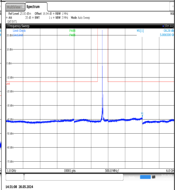
NTVN-N77-3700-3980-PC3-30-25-M-DFT-QPSK-Edge_1RB_Left-1000-6000-Ant1-PASS
