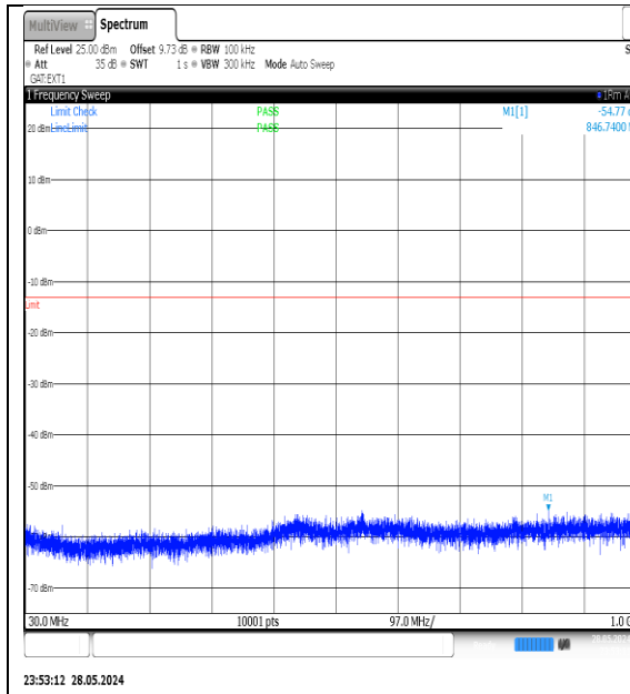
NTNV-N78-3700-3800-PC3-30-90-M-DFT-QPSK- Edge_1RB_Left-30-1000-Ant1-PASS
