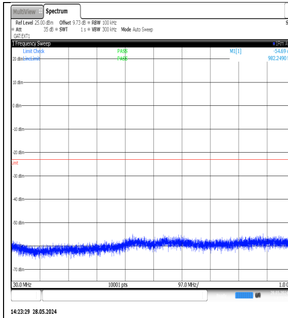
NTNV-N77-3700-3980-PC3-30-20-M-DFT-QPSK- Edge_1RB_Left-30-1000-Ant1-PASS
