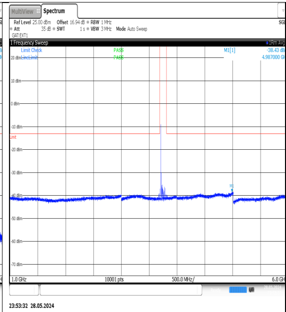
NTNV-N78-3700-3800-PC3-30-90-M-DFT-QPSK- Edge_1RB_Left-1000-6000-Ant1-PASS
