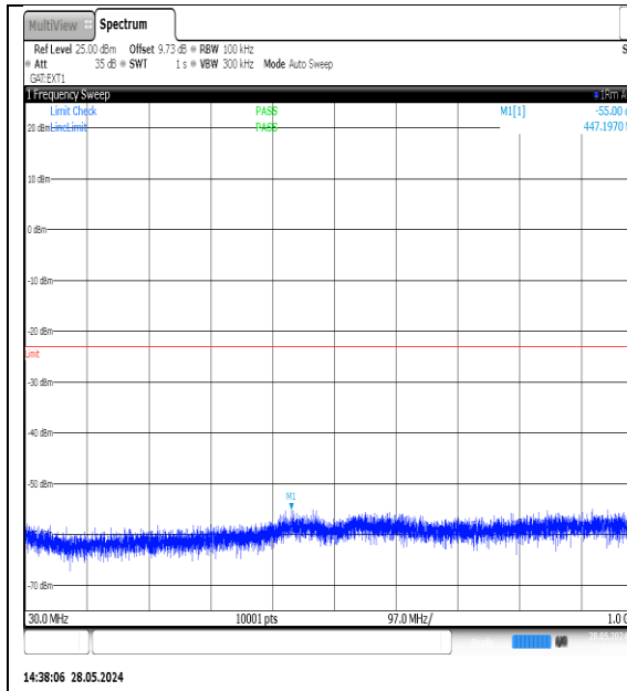
NTVN-N77-3700-3980-PC3-30-30-M-DFT-QPSK-Edge_1RB_Left-30-1000-Ant1-PASS
