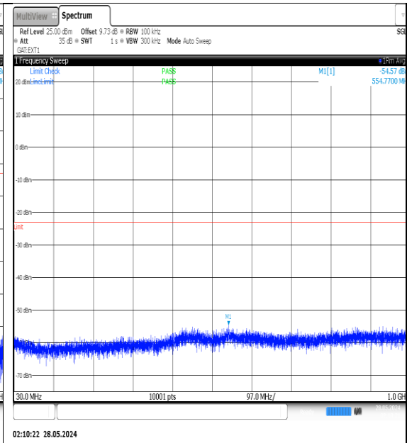
NTNV-N77-3450-3550-PC3-30-50-M-DFT-QPSK-Edge_1RB_Left-30-1000-Ant1-PASS
