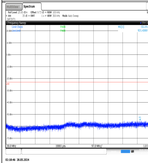
NTVN-N77-3450-3550-PC3-30-60-M-DFT-QPSK-Edge_1RB_Left-30-1000-Ant1-PASS
