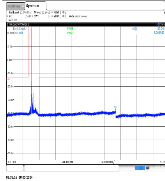
NTNV-N77-3450-3550-PC3-30-80-M-DFT-QPSK- Edge_1RB_Left-3000-6000-Ant1-PASS
