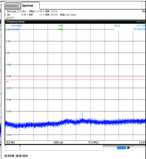
NTNV-N77-3450-3550-PC3-30-90-M-DFT-QPSK-Edge_1RB_Left-30-1000-Ant1-PASS
