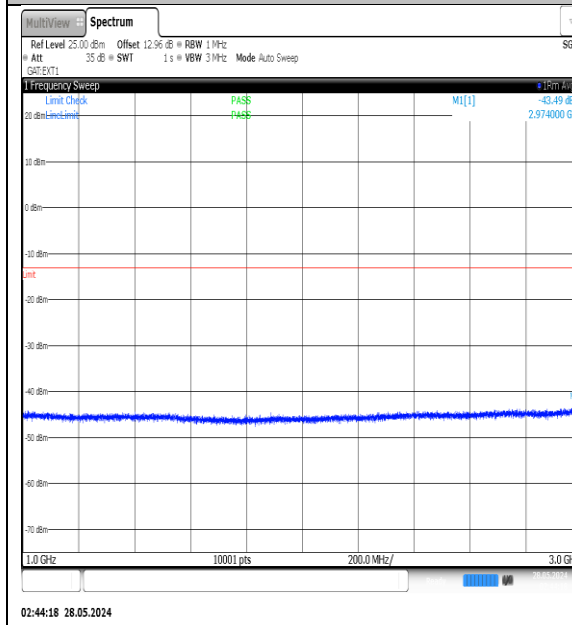
NTNV-N77-3450-3550-PC3-30-90-M-DFT-QPSK-Edge_1RB_Left-1000-3000-Ant1-PASS
