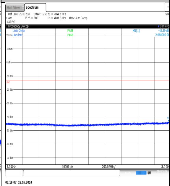
NTVN-N77-3450-3550-PC3-30-60-M-DFT-QPSK-Edge_1RB_Left-1000-3000-Ant1-PASS
