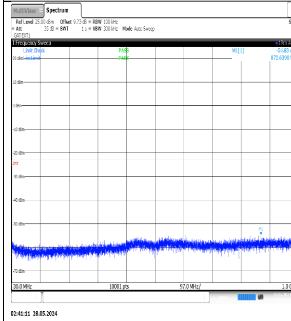
NTNV-N77-3450-3550-PC3-30-90-L-DFT-QPSK-Edge_1RB_Left-30-1000-Ant1-PASS
