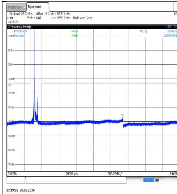
NTVN-N77-3450-3550-PC3-30-60-M-DFT-QPSK-Edge_1RB_Left-3000-6000-Ant1-PASS
