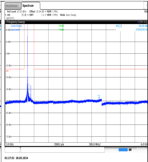
NTNV-N77-3450-3550-PC3-30-70-M-DFT-QPSK-Edge_1RB_Left-3000-6000-Ant1-PASS
