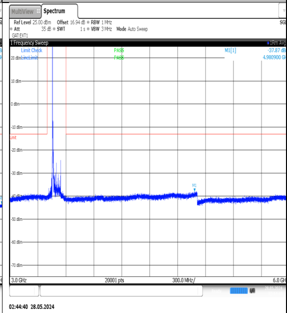
NTNV-N77-3450-3550-PC3-30-90-M-DFT-QPSK-Edge_1RB_Left-3000-6000-Ant1-PASS
