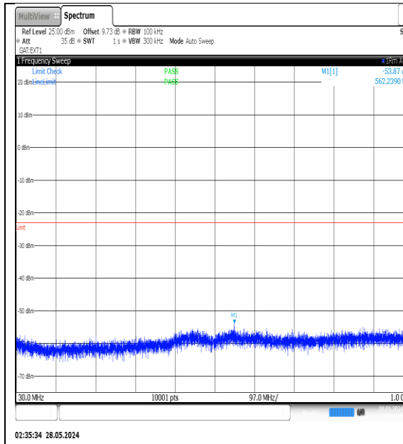
NTNV-N77-3450-3550-PC3-30-80-M-DFT-QPSK- Edge_1RB_Left-30-1000-Ant1-PASS
