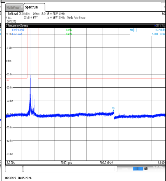
NTNV-N77-3450-3550-PC3-30-80-L-DFT-QPSK- Edge_1RB_Left-3000-6000-Ant1-PASS
