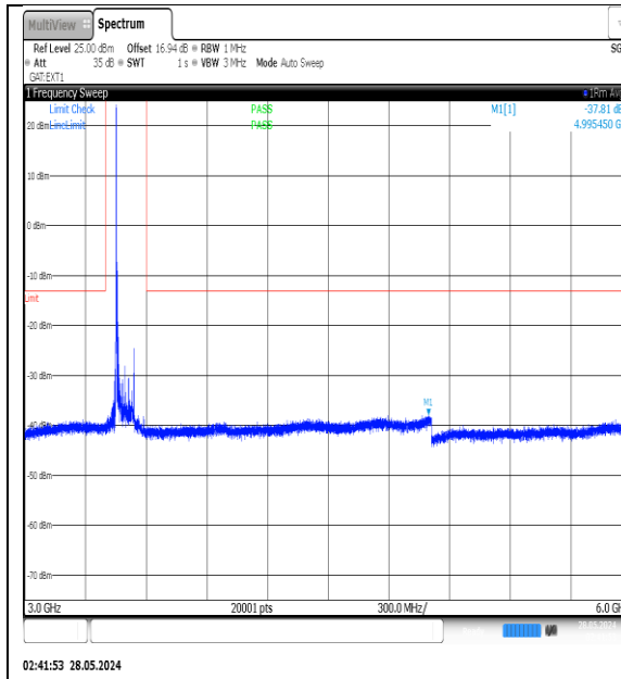
NTNV-N77-3450-3550-PC3-30-90-L-DFT-QPSK- Edge_1RB_Left-3000-6000-Ant1-PASS
