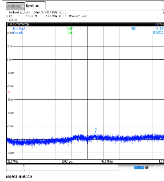
NTNV-N77-3450-3550-PC3-30-50-L-DFT-QPSK-Edge_1RB_Left-30-1000-Ant1-PASS
