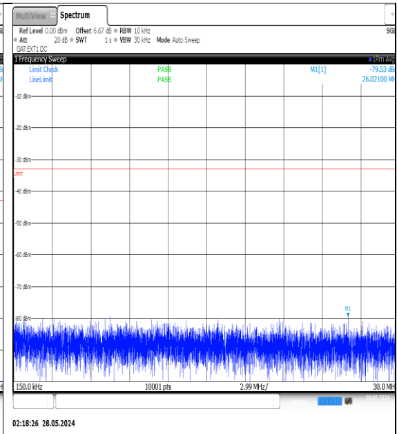
NTVN-N77-3450-3550-PC3-30-60-M-DFT-QPSK-Edge_1RB_Left-0.15-30-Ant1-PASS
