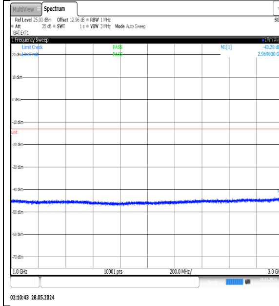
NTNV-N77-3450-3550-PC3-30-50-M-DFT-QPSK-Edge_1RB_Left-1000-3000-Ant1-PASS
