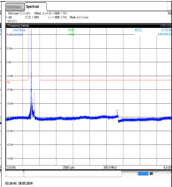
NTNV-N77-3450-3550-PC3-30-60-L-DFT-QPSK- Edge_1RB_Left-3000-6000-Ant1-PASS
