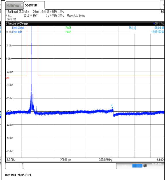
NTNV-N77-3450-3550-PC3-30-50-M-DFT-QPSK-Edge_1RB_Left-3000-6000-Ant1-PASS
