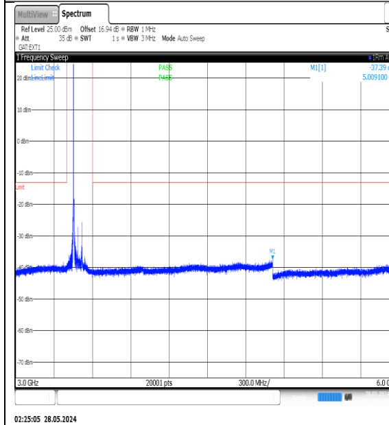
NTNV-N77-3450-3550-PC3-30-70-L-DFT-QPSK- Edge_1RB_Left-3000-6000-Ant1-PASS
