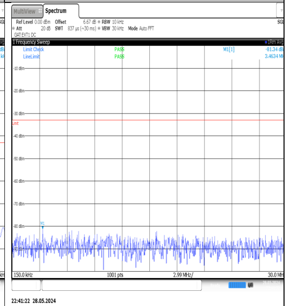
NTVN-N78-3700-3800-PC3-30-15-L-DFT-QPSK-Edge_1RB_Left-0.15-30-Ant1-PASS
