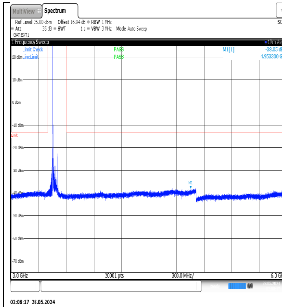
NTNV-N77-3450-3550-PC3-30-50-L-DFT-QPSK- Edge_1RB_Left-3000-6000-Ant1-PASS
