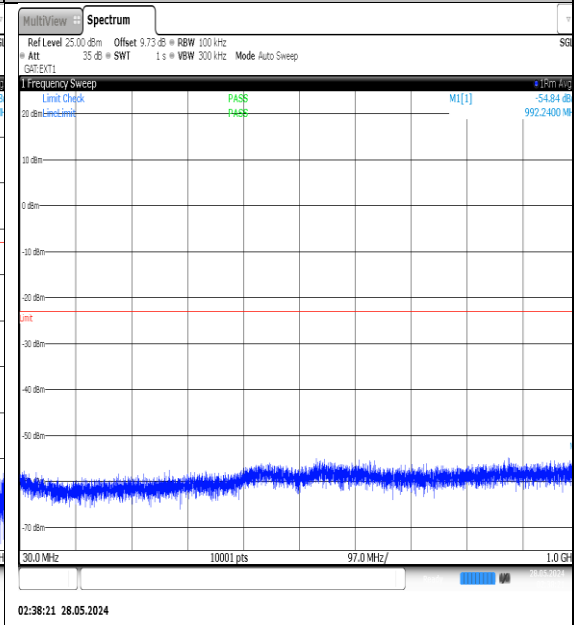
NTVN-N77-3450-3550-PC3-30-80-H-DFT-QPSK-Edge_1RB_Left-30-1000-Ant1-PASS
